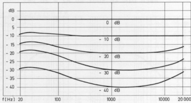
Fig. 5 Wirkungsweise der physiologischen Lautstärkeregelung 0 dB = Lautstärkereglers offen
