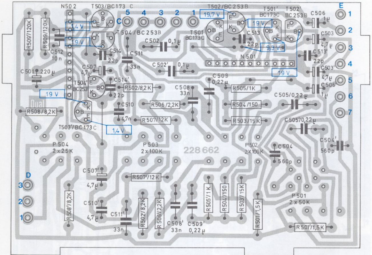
Fig. 9 Regelverstärker 230 606 (Leiterseite)
