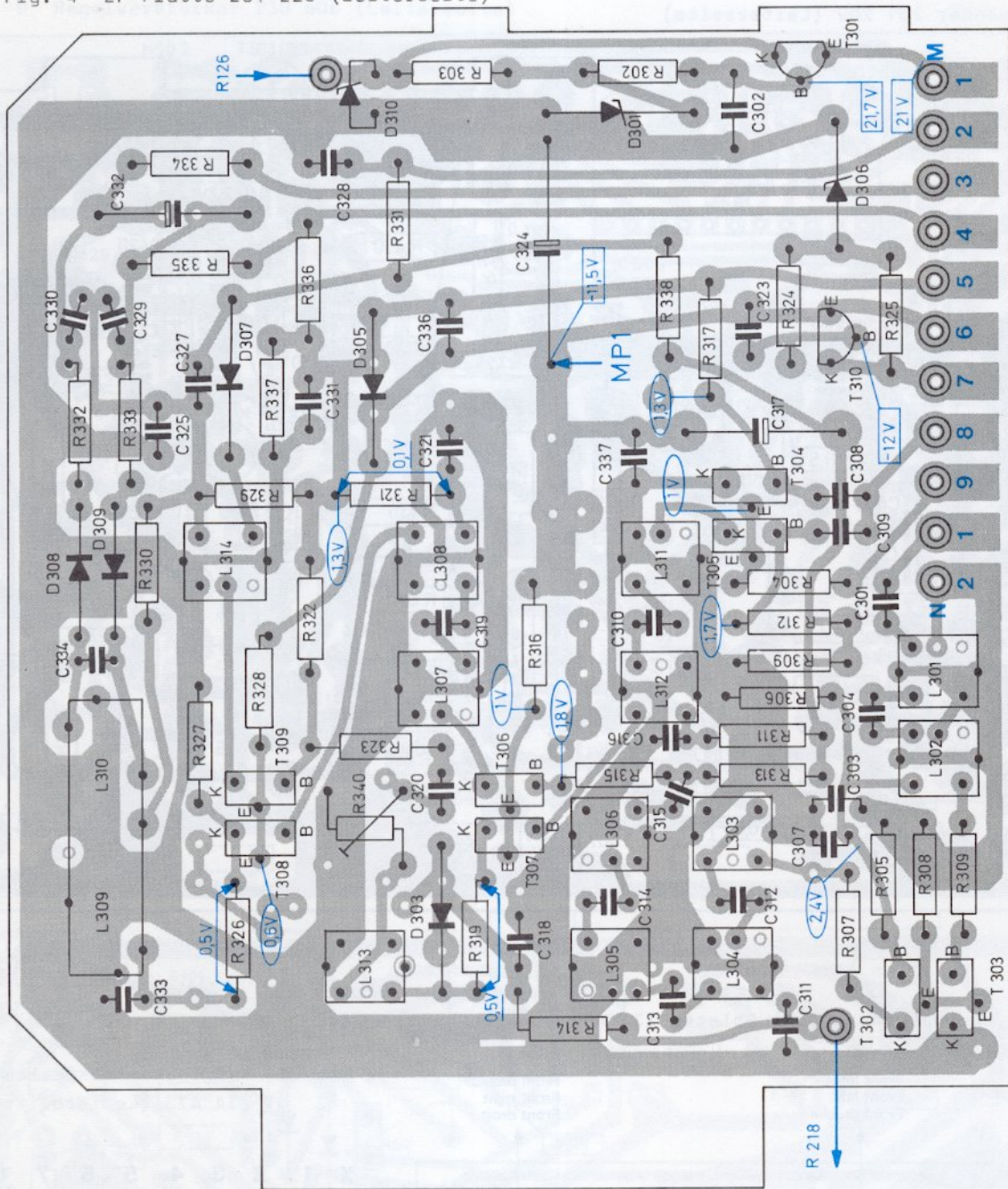
Fig. 5 Vorverstärker 227 746 (Leiterseite)
