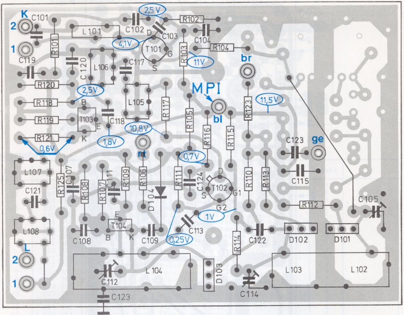
Fig. 11 UKW-Teil 234 211 (Leiterseite)
