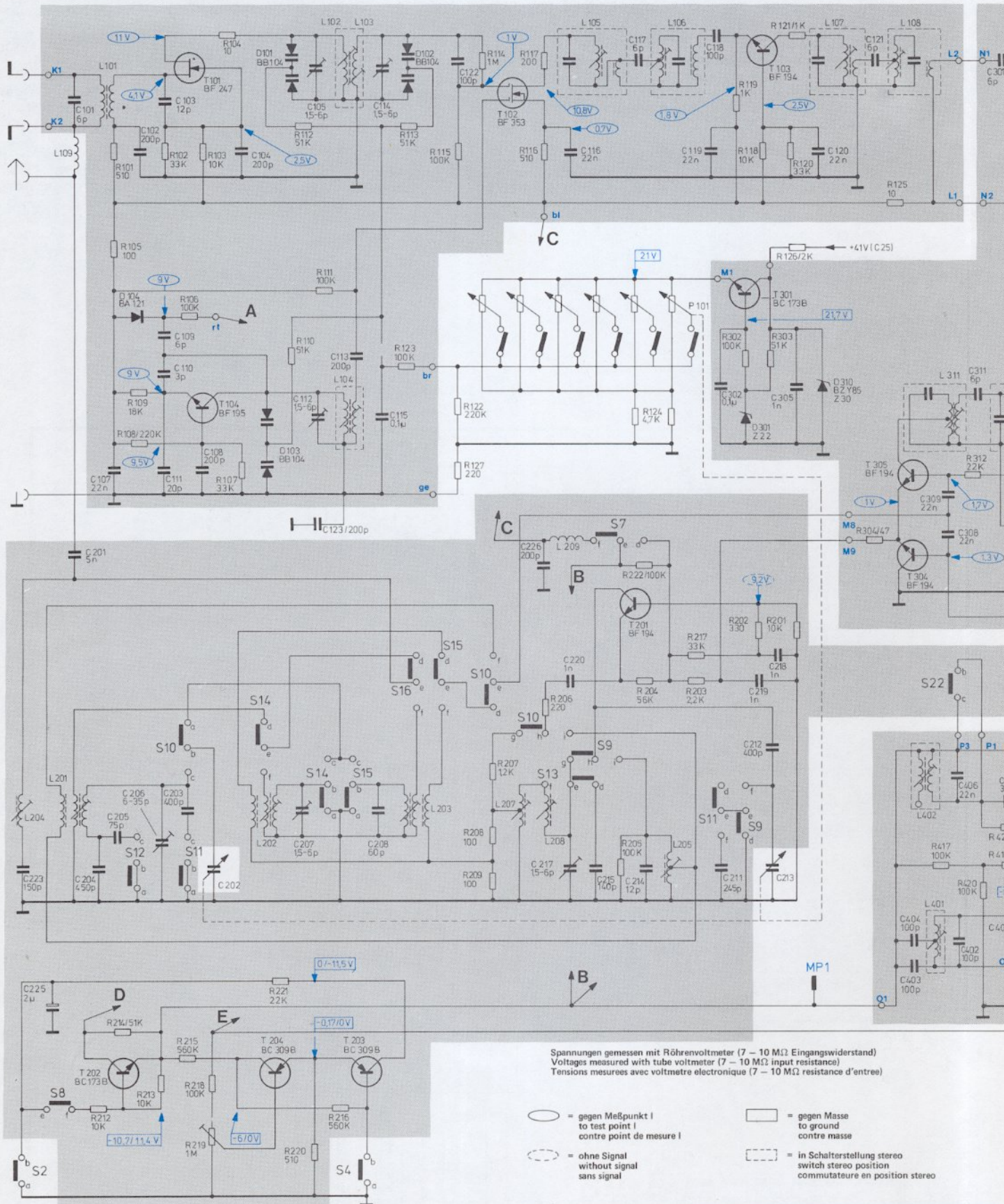
Fig. 2 Schaltbild HF
