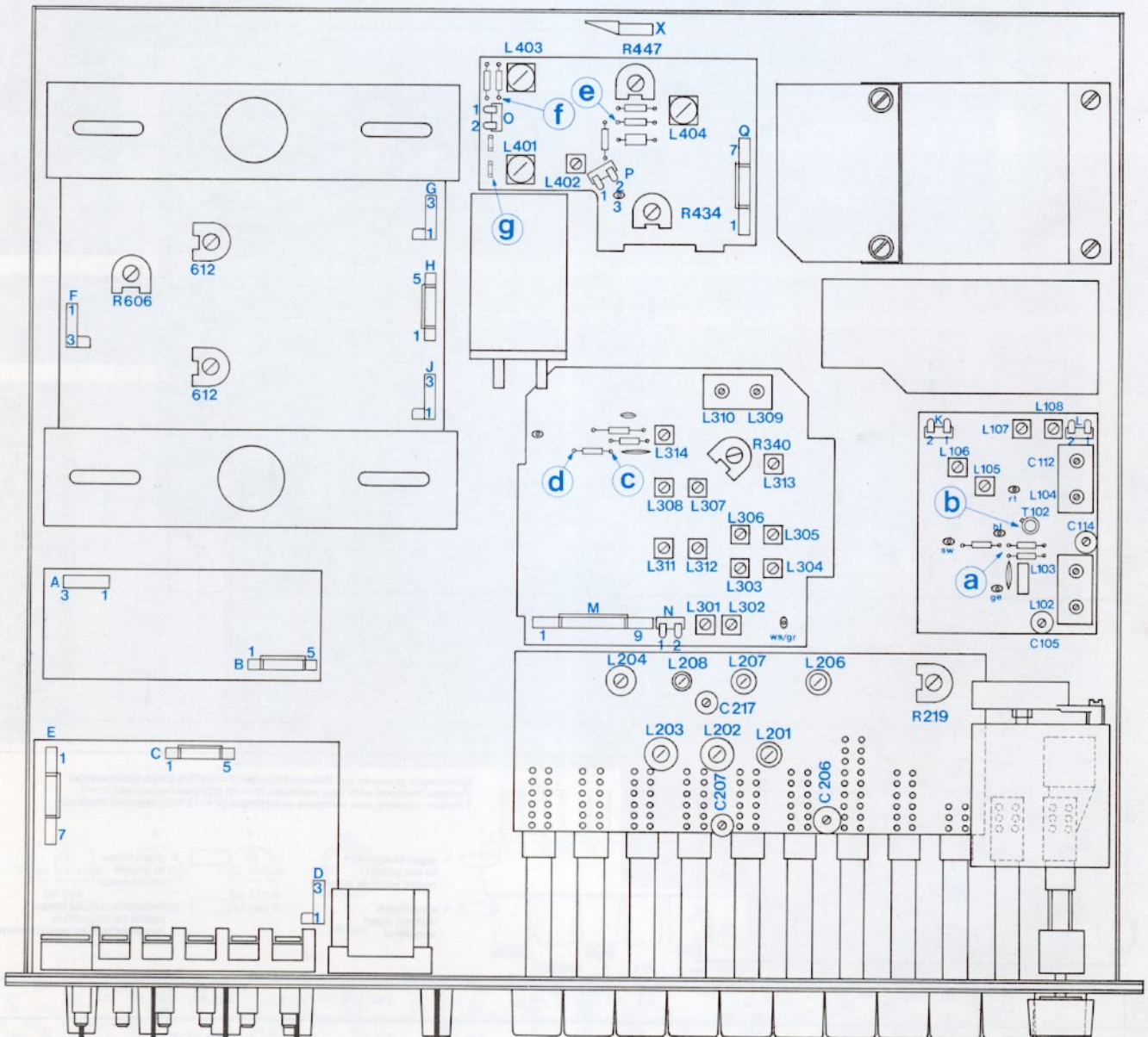
Fig. 1 Abgleichpositionen und Lageplan der Steckverbindungen
