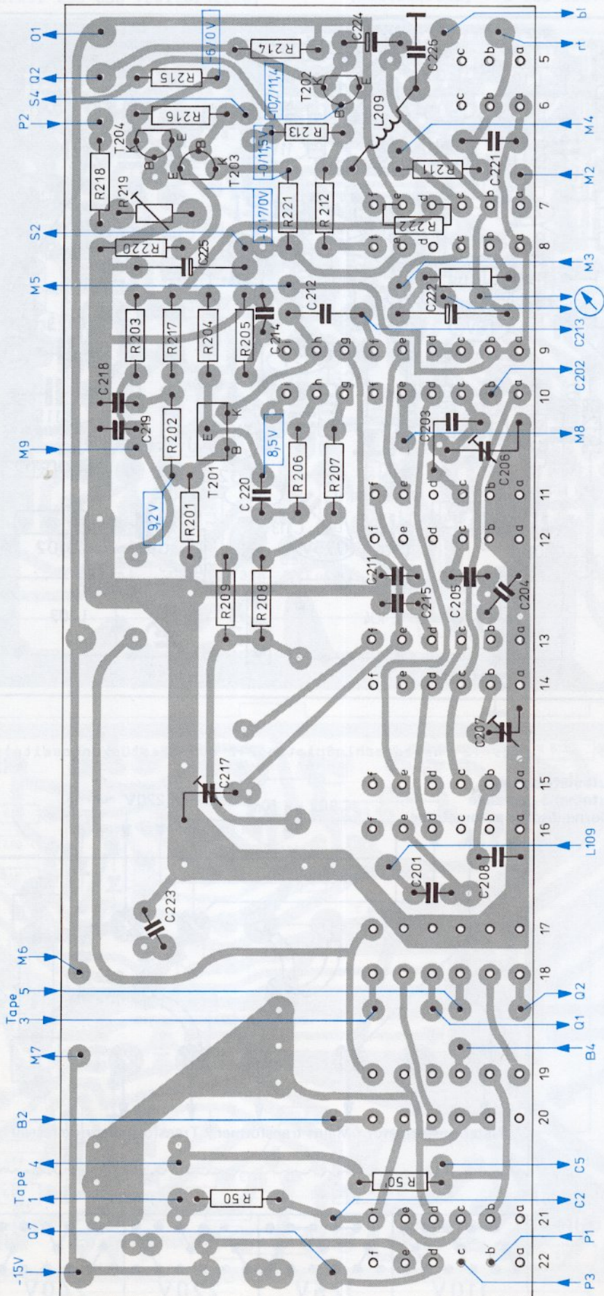
Fig. 13 AM-HF-Teil 231 206 (Leiterseite)
