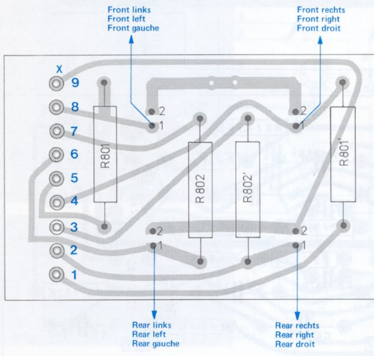
Fig. 7 Lautsprecheranschlußplatte 234 475 (Leiterseite)
