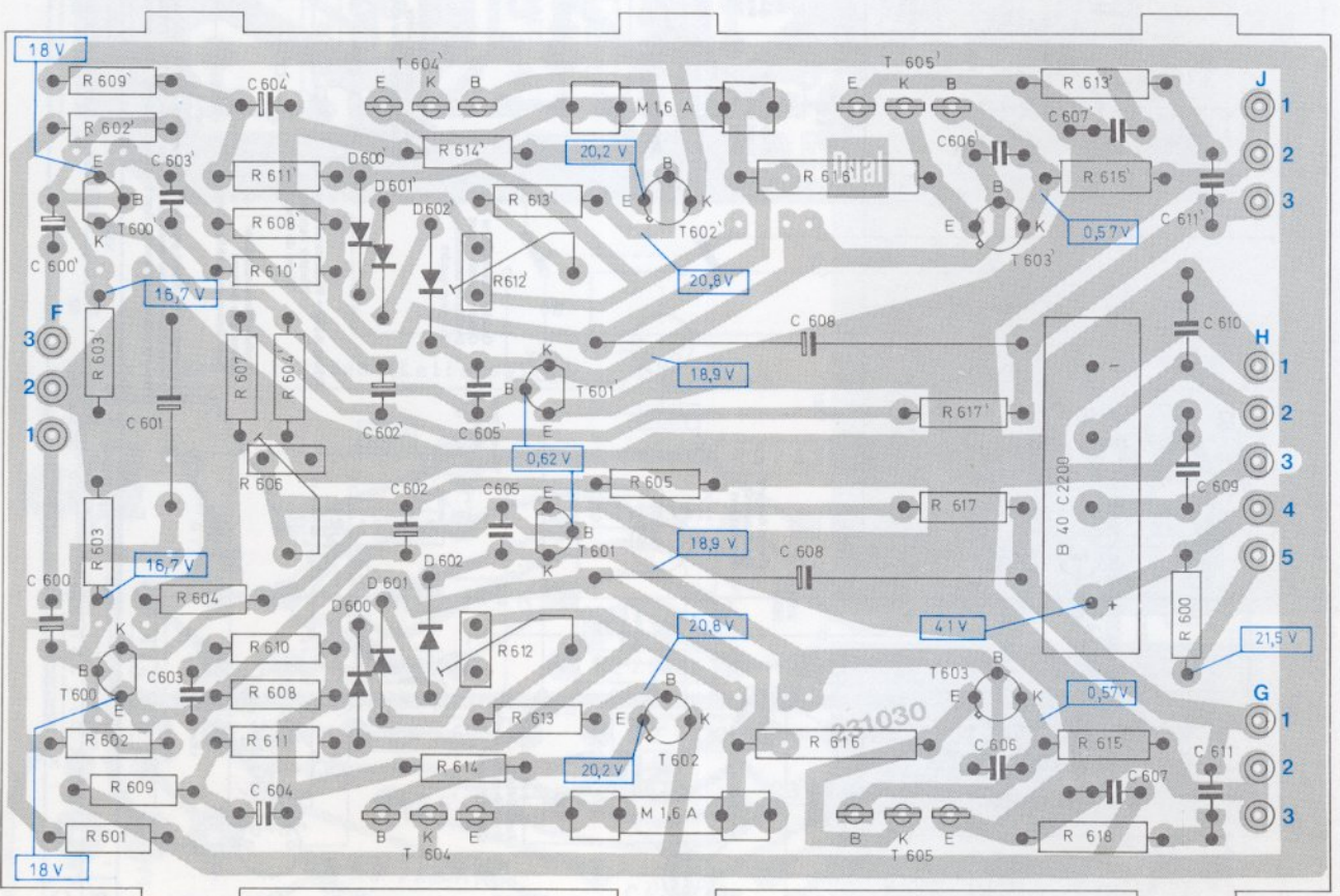
Fig. 10 Endverstärker 234 147 (Leiterseite)
