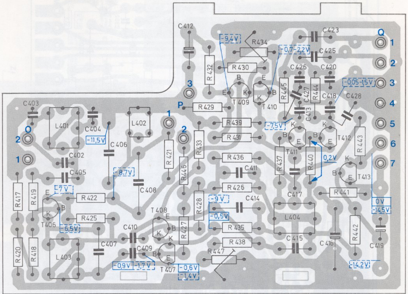
Fig. 6 Decoder 231 209 (Leiterseite)
