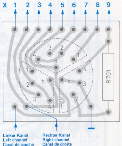
Fig. 8 Betriebsartenschalterplatte 234 473 (Leiterseite)
