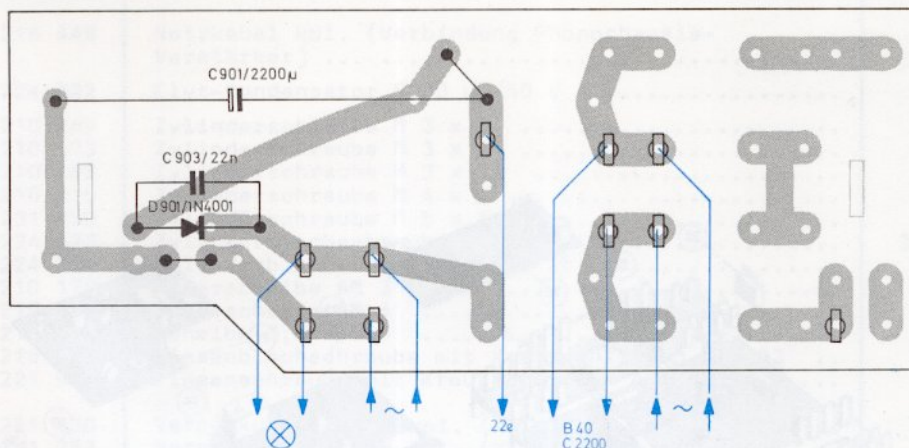
Fig. 14 Gleichrichterplatte 231 217 (Leiterseite)
