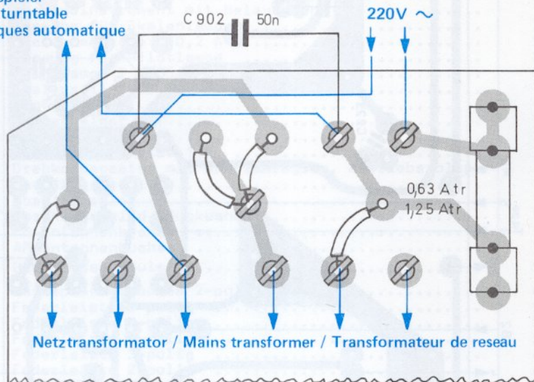
Fig. 12 Netzanschlußplatte 212 600 (Bestückungsseite)
