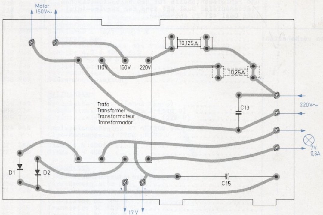
Fig. 3 Anschlußplatte 234 139 (Leiterseite)
