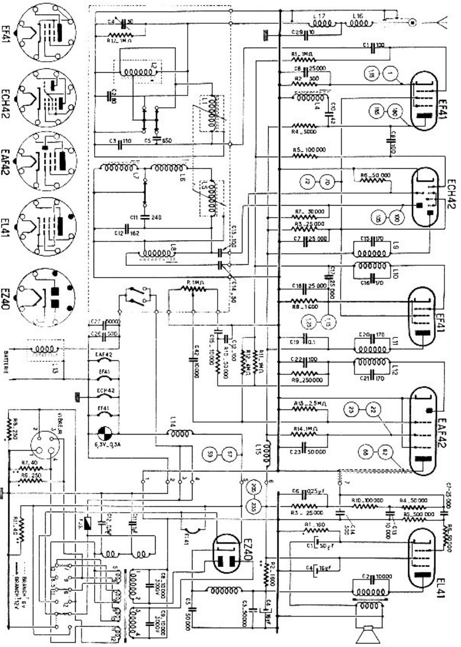
Schéma général du récepteur D1935V 13 modèle 1952
