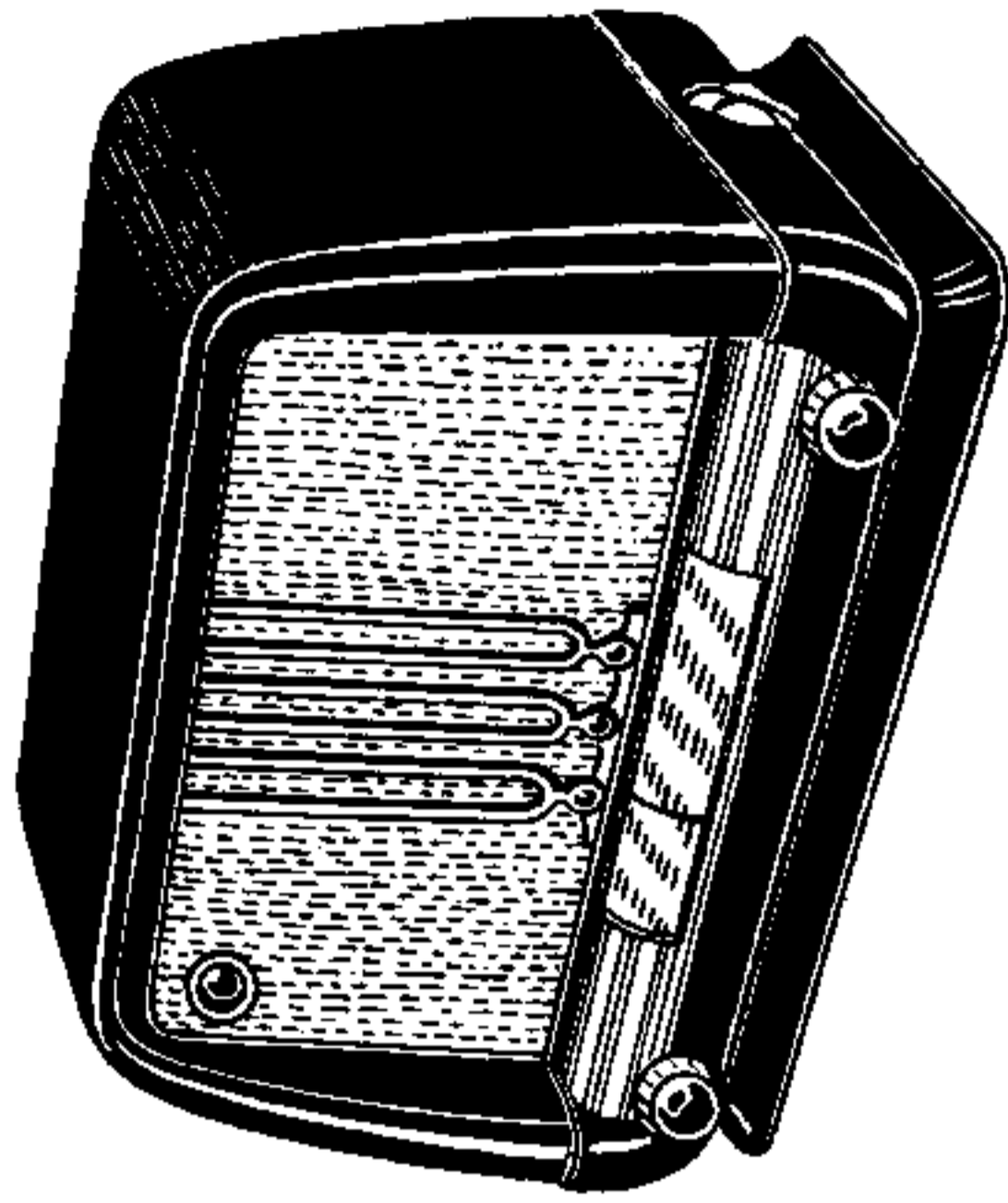
Aspect extérieur du récepteur L026Z.
