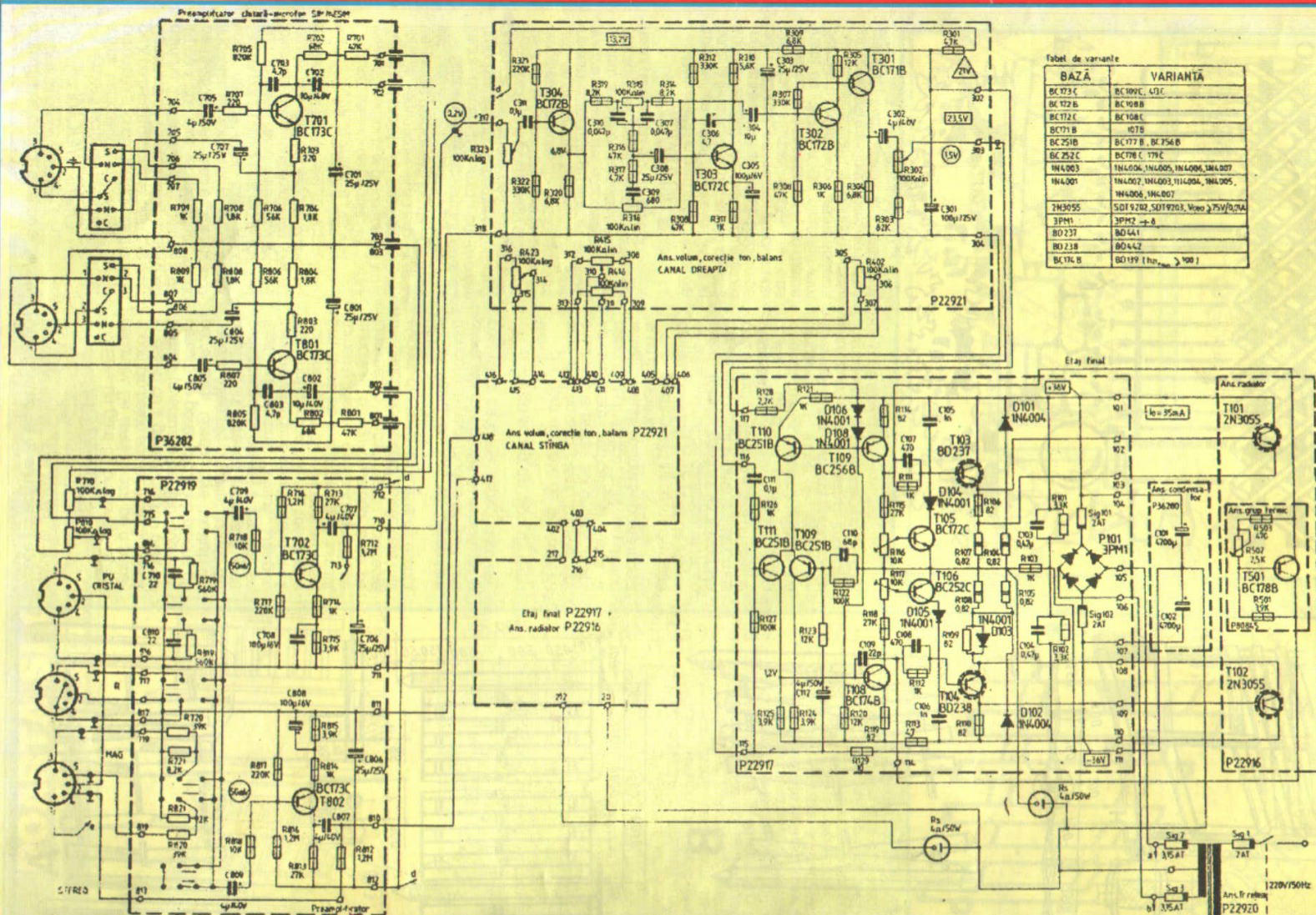
SCHEMA ELECTRICA A AMPLIFICATORULUI AS 2050 P11528-000
