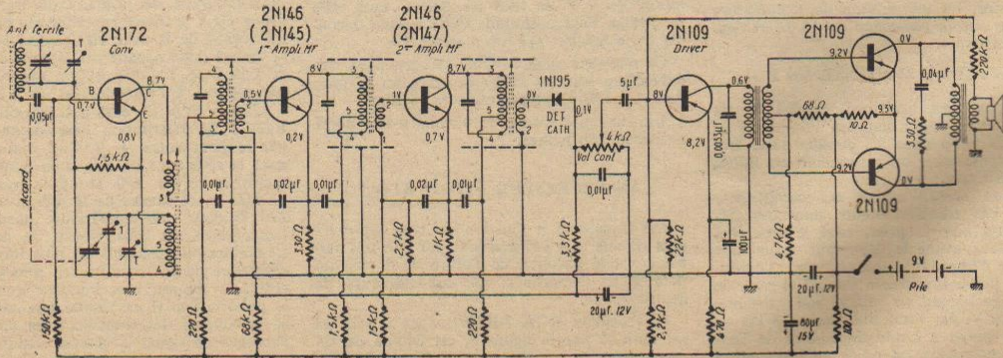
FIG. 10. — Récepteur Emerson 855
