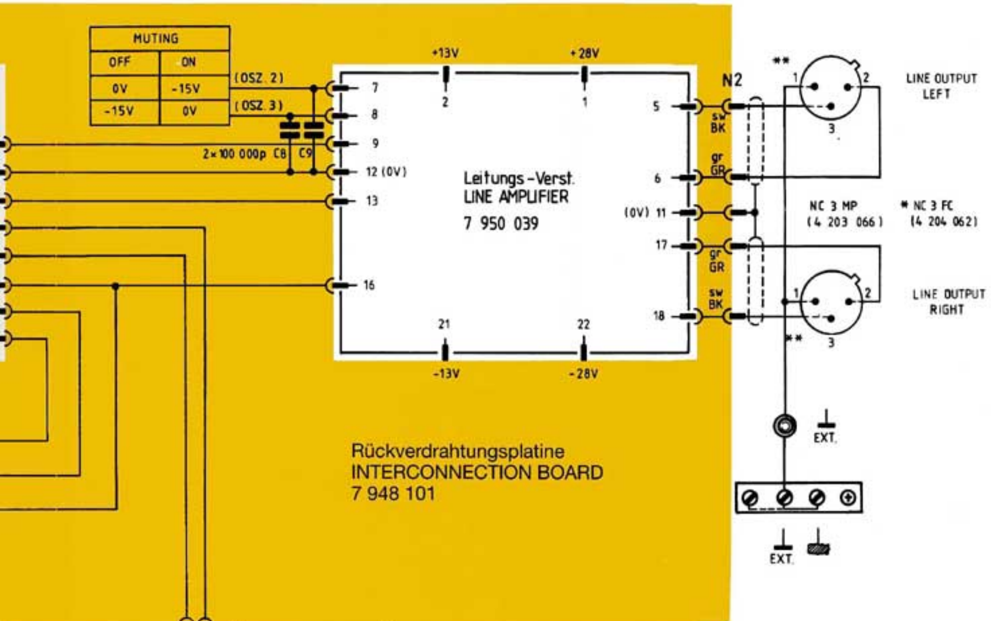
NF Blockschaltbild EMT 948 AUDIO BLOCK DIAGRAM
