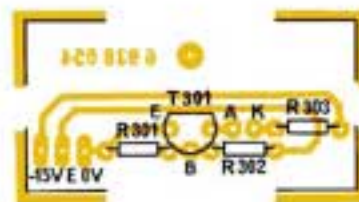
Sync-Anzeige SYNC INDICATOR 7 938 054
