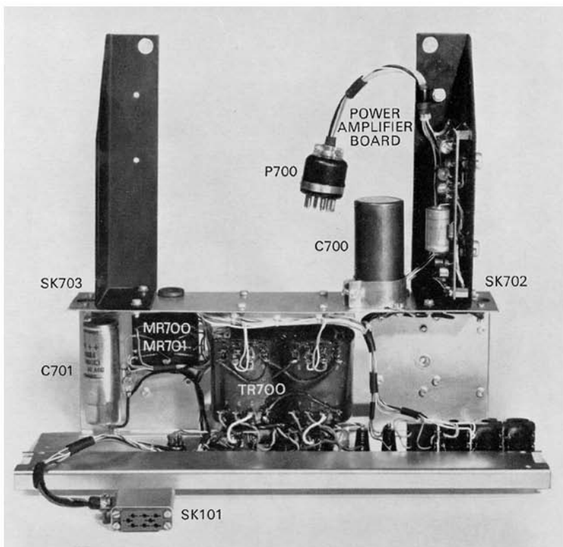
FIG. 30. MONO POWER UNIT
