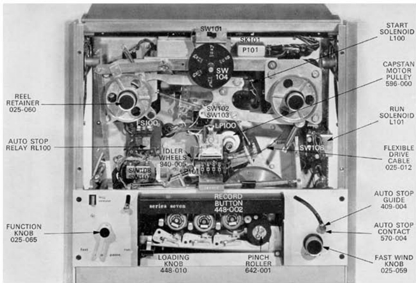
FIG. 20. DECK MECHANICS
