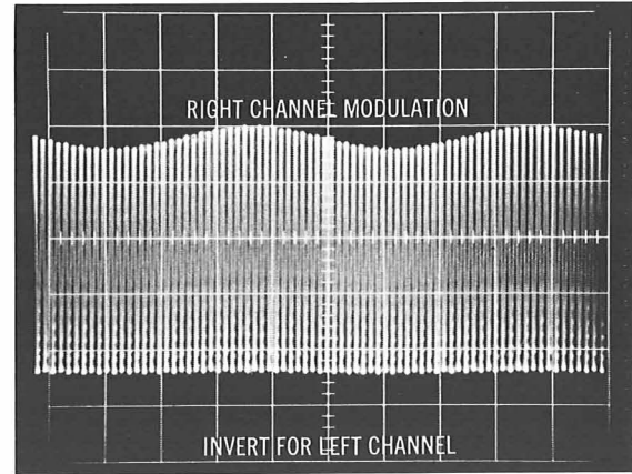
MPX OUTPUT
