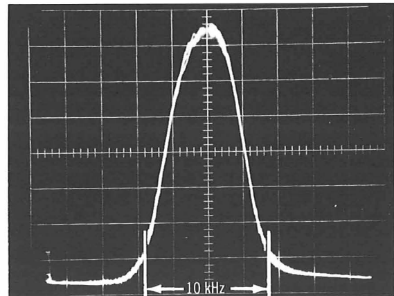
AM IF
