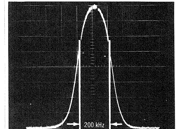
FM IF
