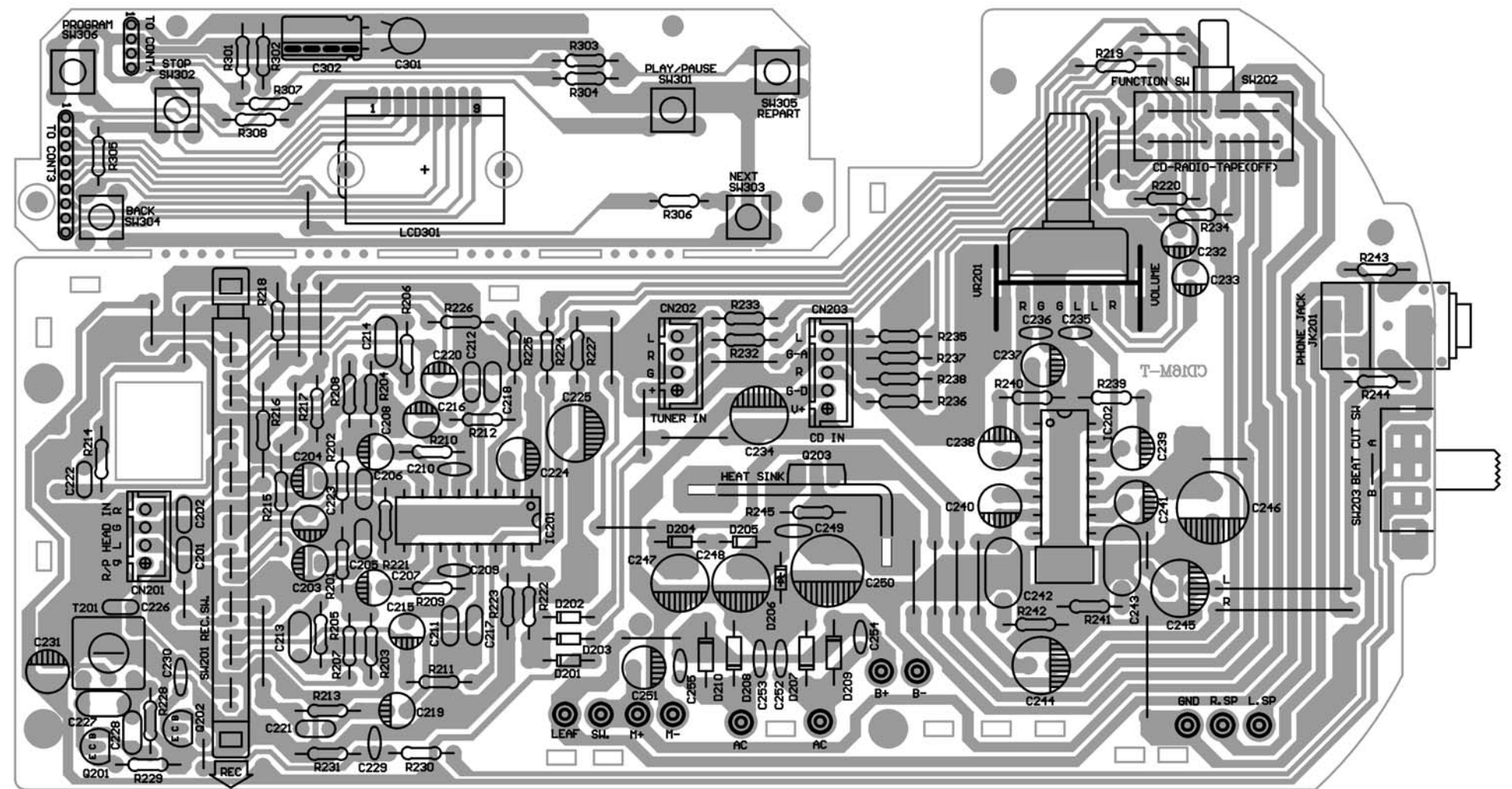
PLACA DE CONTROLE DA UNIDADE ÓPTICA
