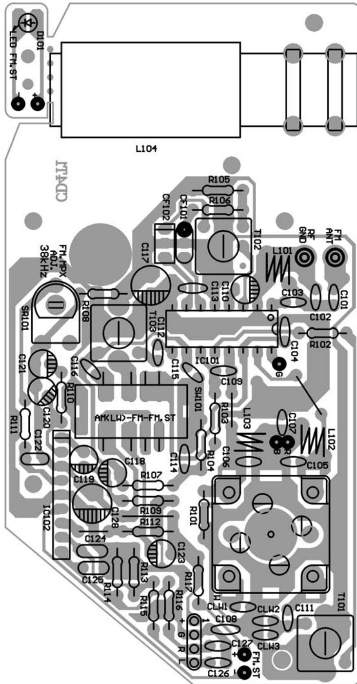
PLACA DO RÁDIO
