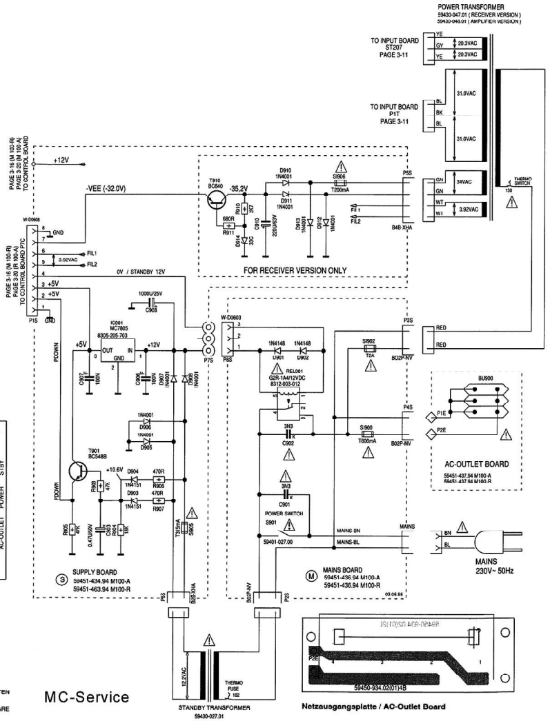
Spannungsversorgungsplatte / Supply Board
