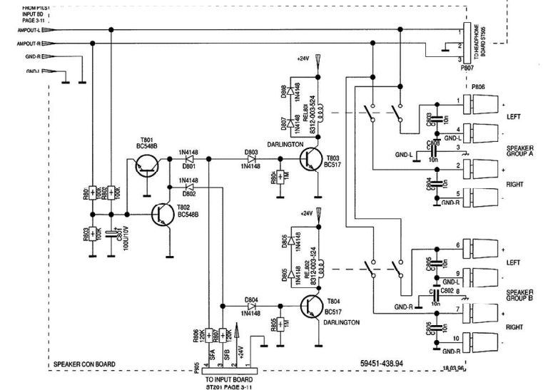
NF-Ausgangsplatte / AF Output Board
