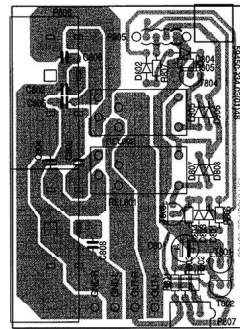
NF-Ausgangsplatte / AF Output Board
