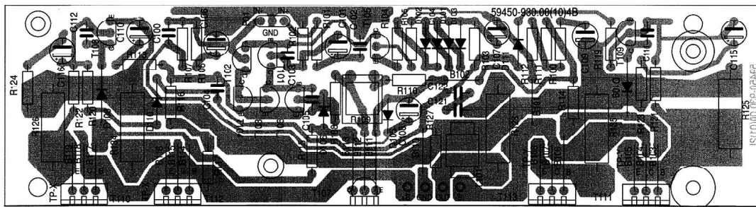
Verstärkerplatte / Amplifier Board
