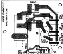
Netzteilplatte / Mains Board
