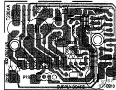
Spannungsversorgungsplatte / Supply Board
