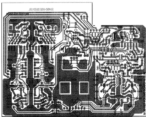
Lautstärkeregerplatte / Volume Control Board
