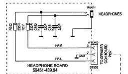
Kopfhörerbuchsenplatte Headphone Socket Board
