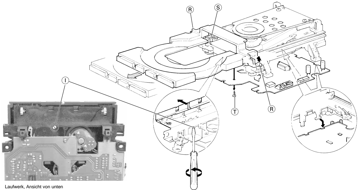
Laufwerk, Ansicht von unten Drive mechanism, bottom view
