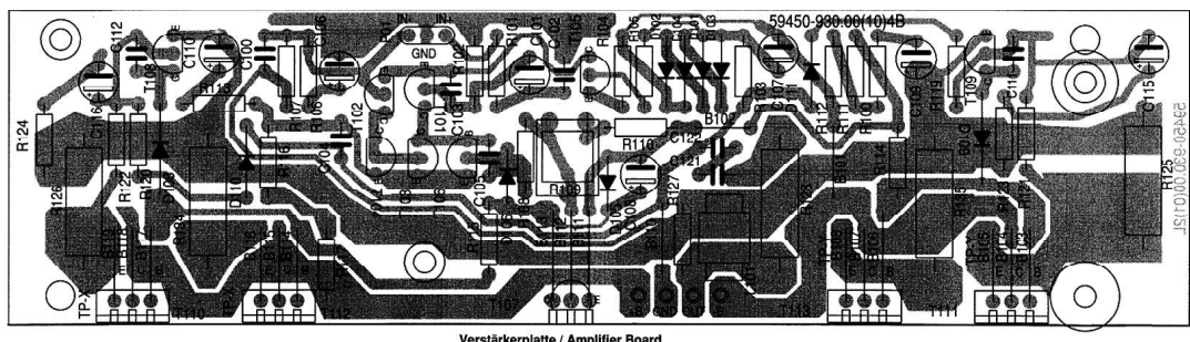
Verstärkerplatte / Amplifier Board
