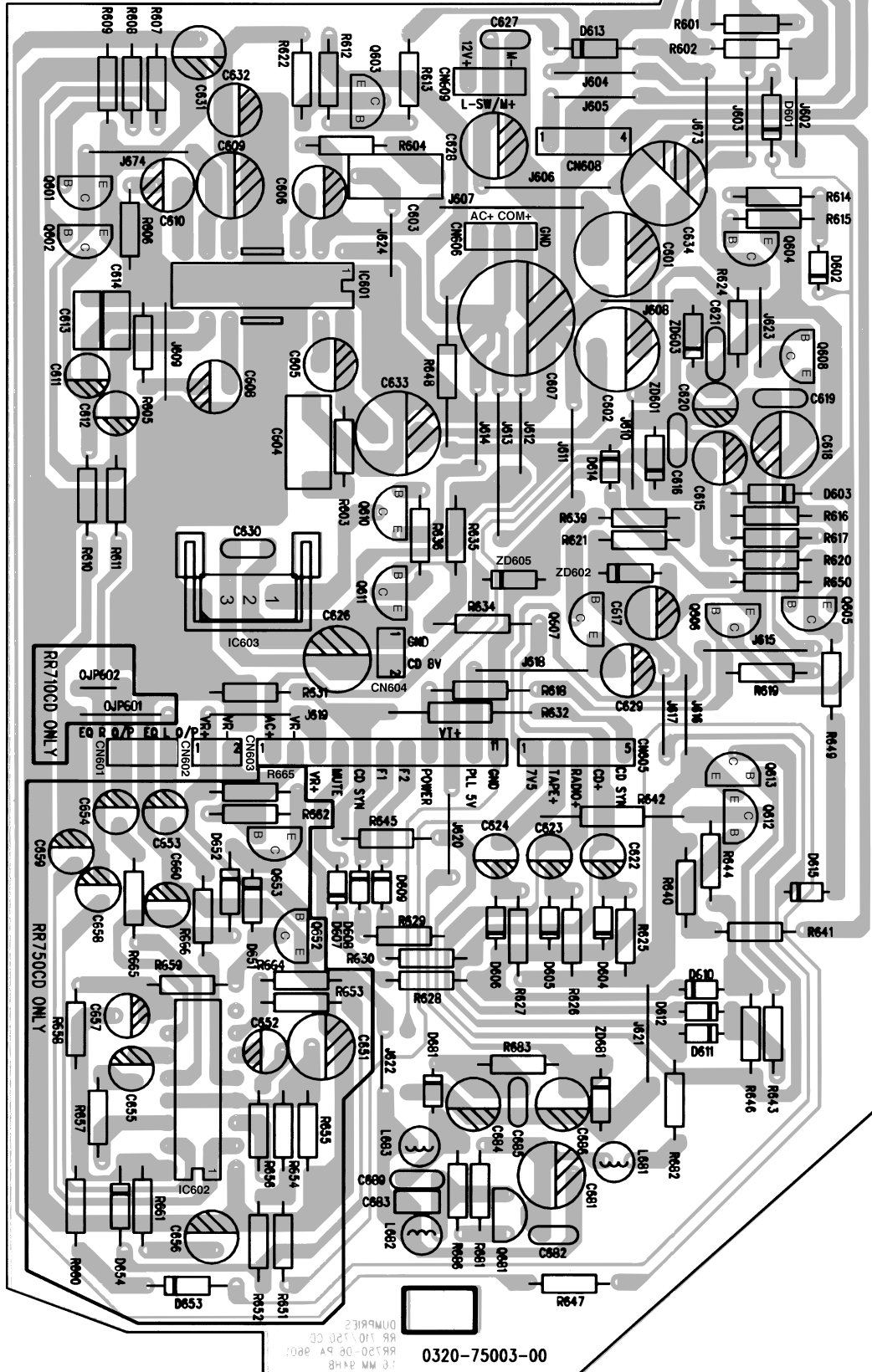
AF / Power Board Bestückungsseite / Component Side
