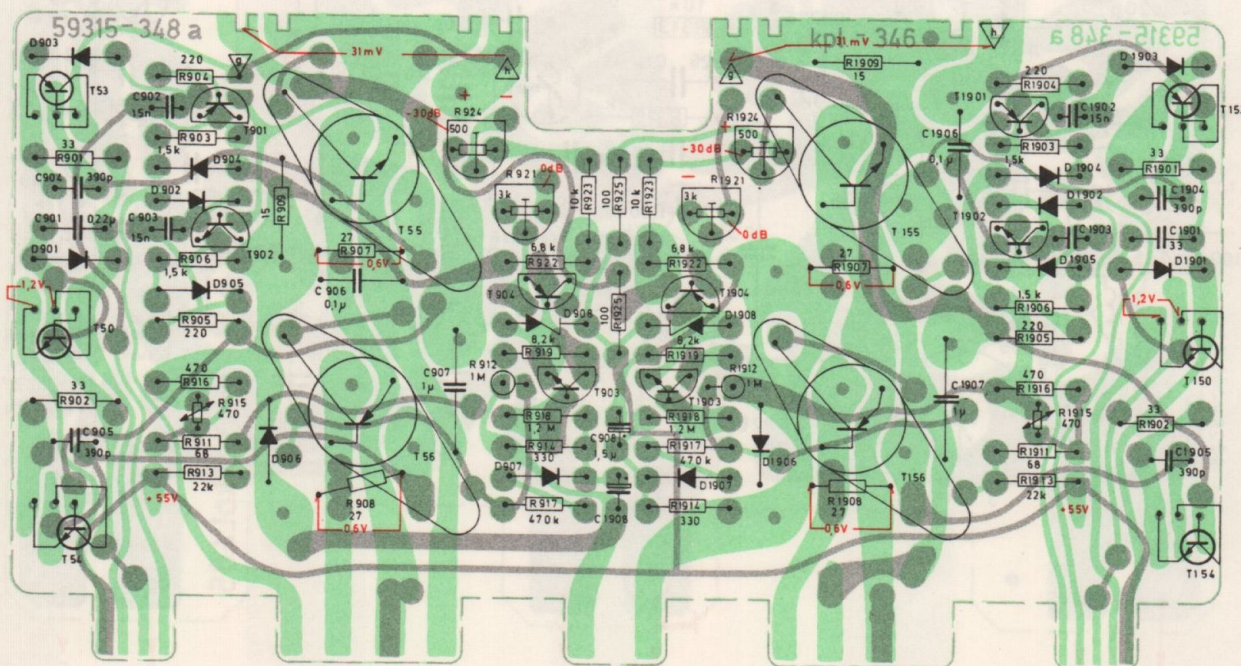
Endstufen - Platte RC 1040
