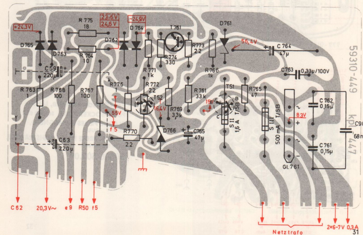
Netzteilplatte, Lötseite MAINS UNIT PRINTED BOARD, SOLDER SIDE PLAQUE SECTEUR, COTE SOUDURES PIASTRA SEZIONE RETE, LATO SALDATURE 59310-076.00
