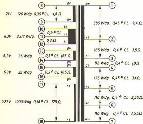
Netztrafo BV 9007—503
