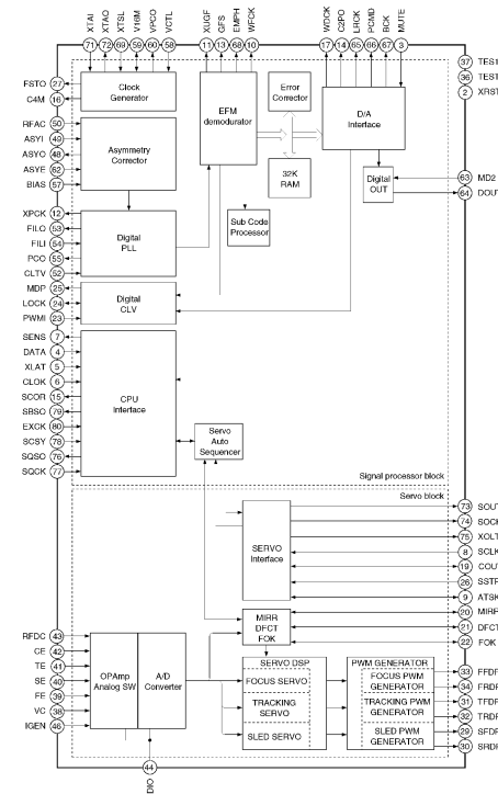
IC701 CXD2068Q
