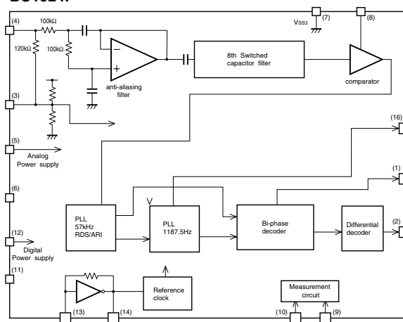
IC103 BU1924F
