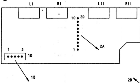
(D) LS-BUCHSEN-PLATTE 59351-046.00
