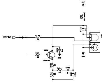
SPDIF OUT
