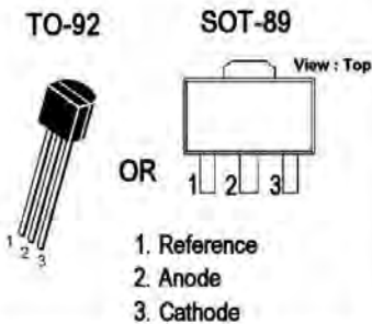
KIA431B
