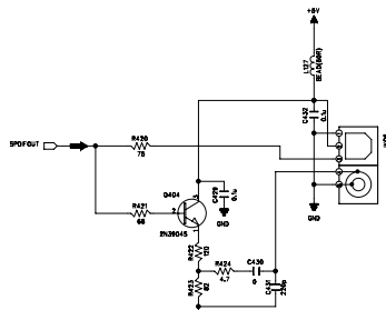
SPDIF OUT
