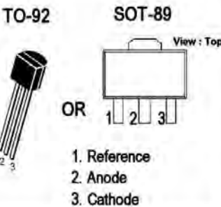
KIA431B
