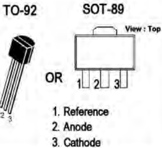
KIA431B
