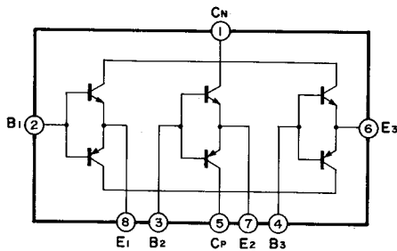
IC103 : STA341M Transistor Array
