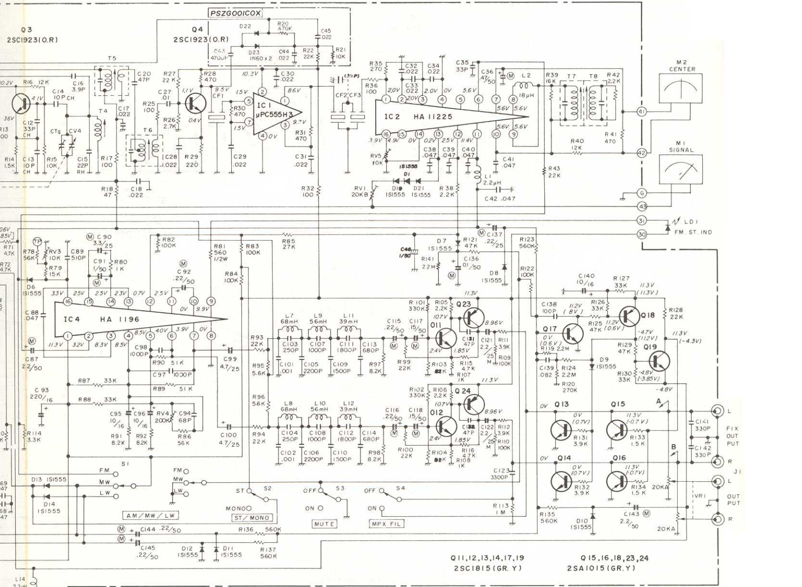
Q15,16,18,23,24 2SA1015 (GR. Y)
