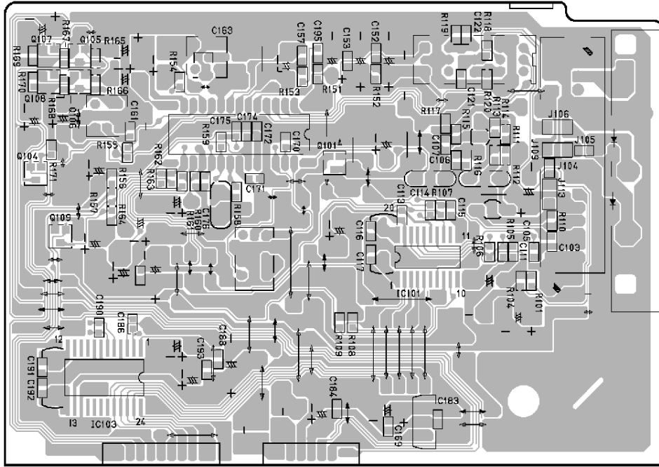
TU PWB
