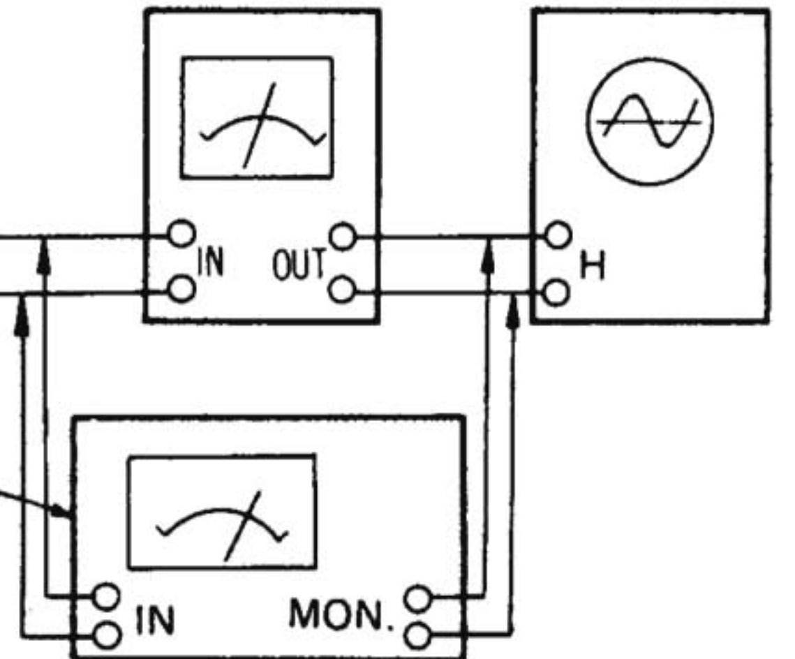
AC Voltmeter Wechselspannungsmesser Voltmètre à courant alternatif
