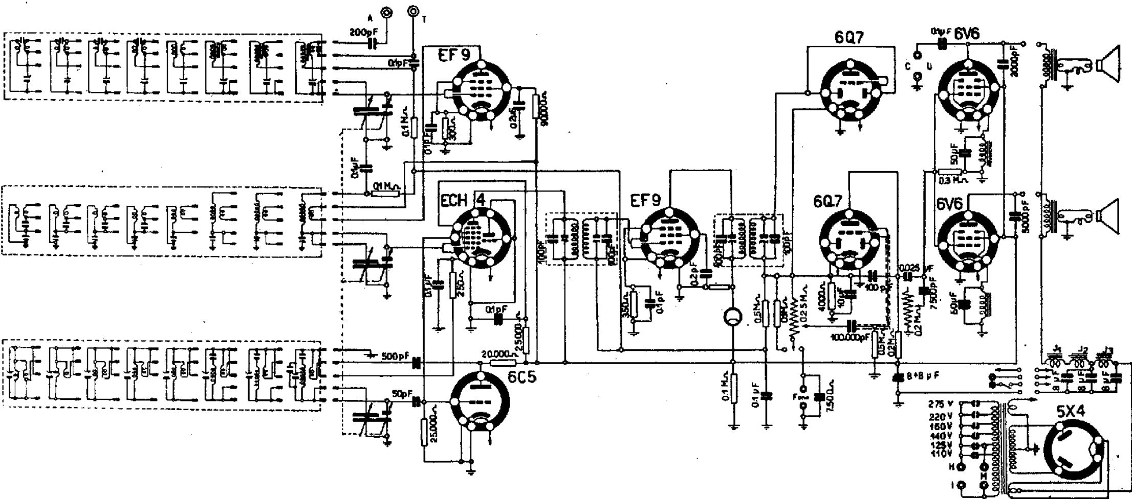
IMCA RADIO - Mod. IF 92S SERIE MULTIGAMMA IV - Una gamma onde lunghe, due gamme onde medie, quattro gamme onde corte. Conversione di frequenza con ECH4 mescolatrice e 6C5 oscillatrice separata. Potenza d'uscita: 12 watt. Media frequenza: 467 kc.
