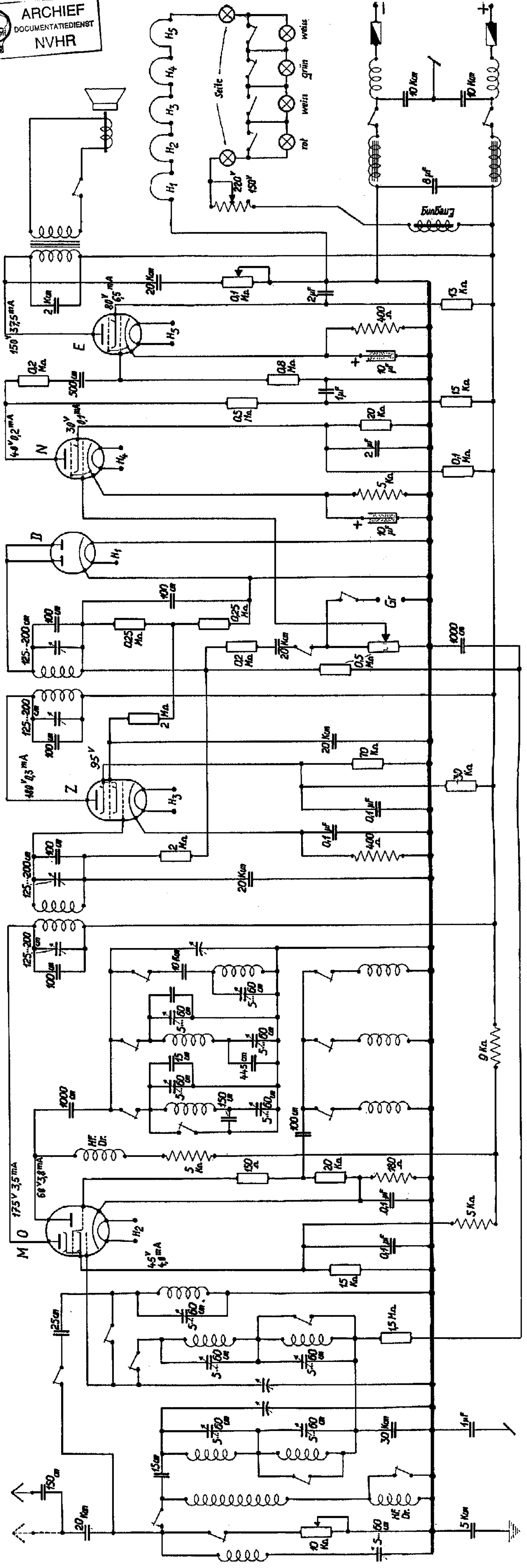
Abb. 551. Lorenz, Supercelohet Senior KG, Gleichstrom, 2 Vorkreise 4 Zwischenfrequenzkreise, Gruppe 57
