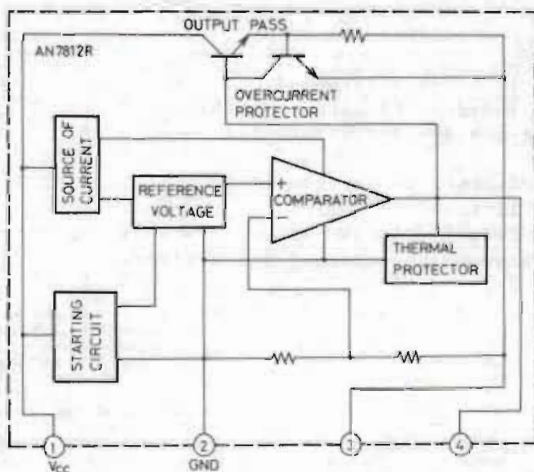
IC103 : AN7812R (Regulator)
