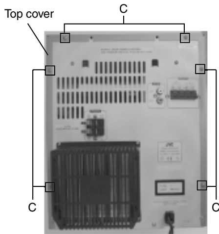
CA-MXKA3A Fig.4 (A)
