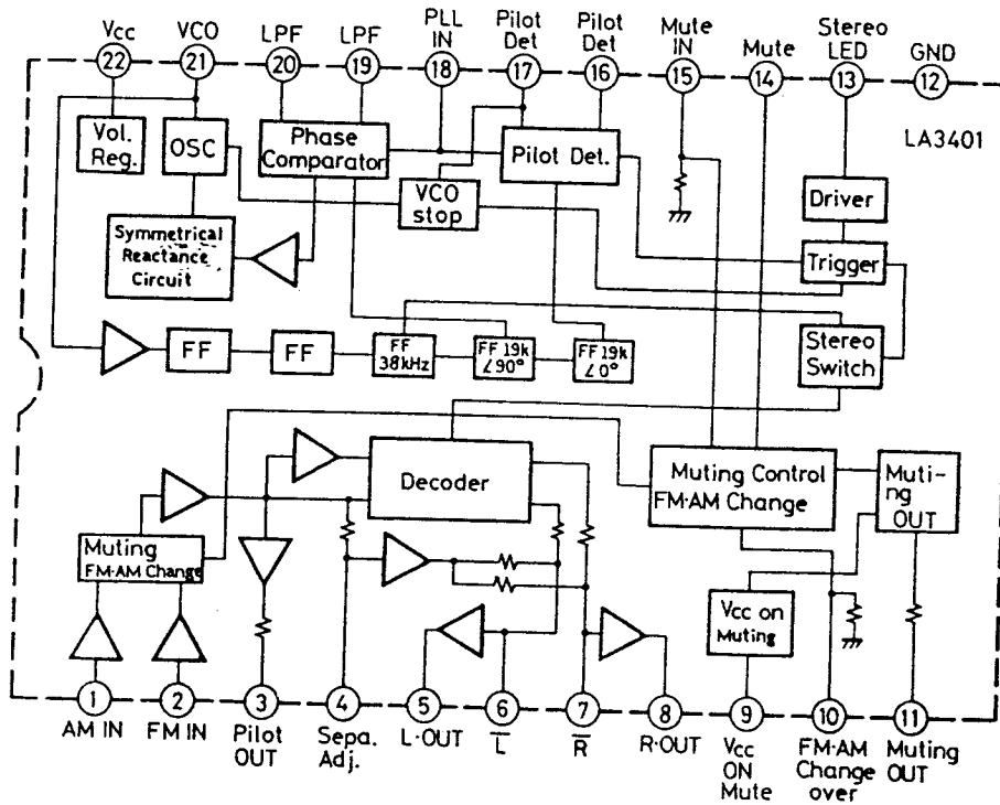
IC171: LA3401
