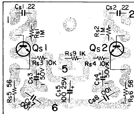
Qs1, 2 2SC458LG (D)
