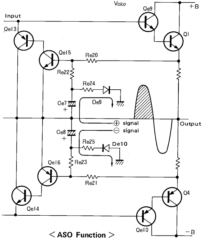
< ASO Function >
