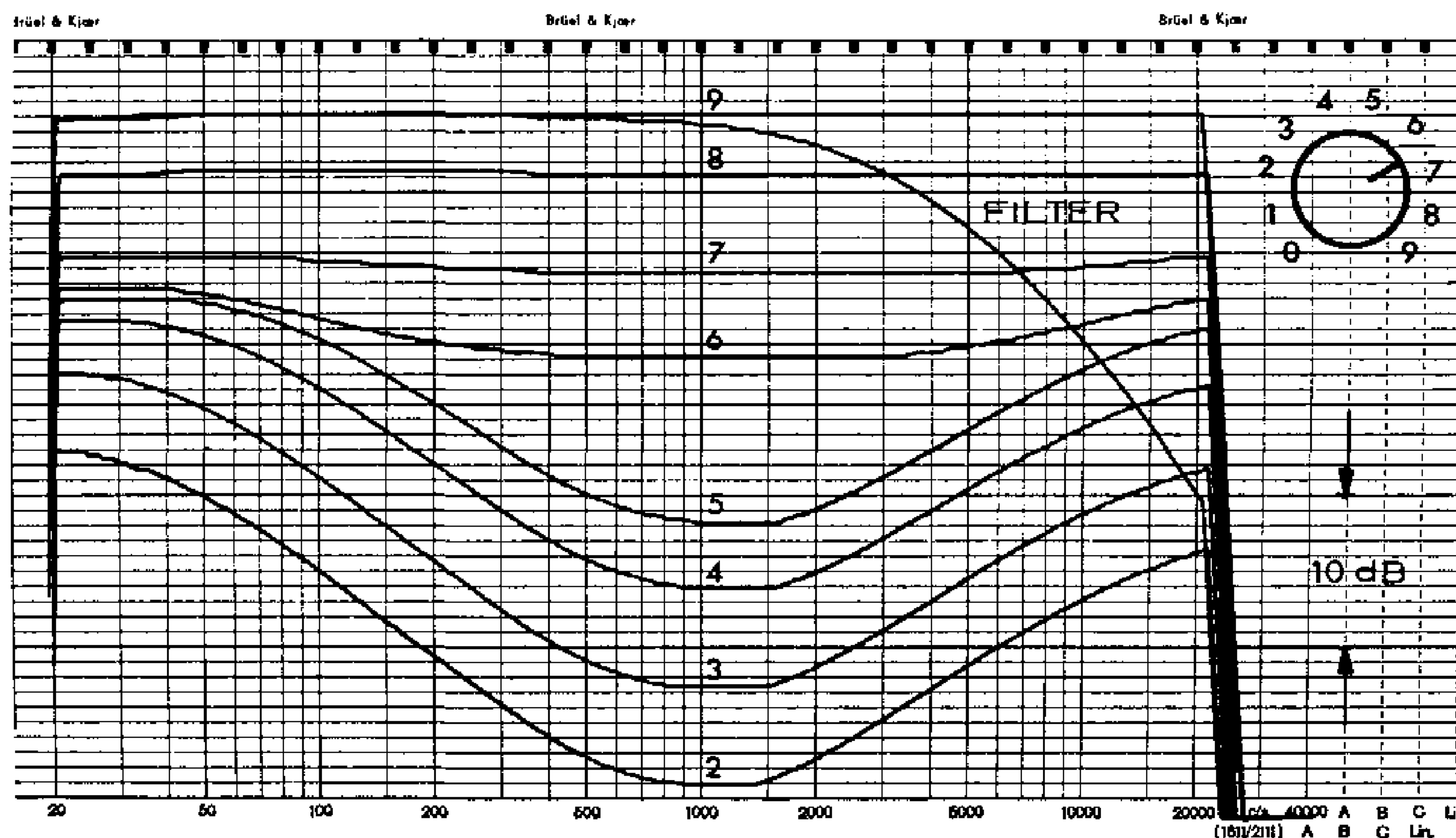
Frequenzgang Lautstärkereglern (Contour) und Höhenfilter
