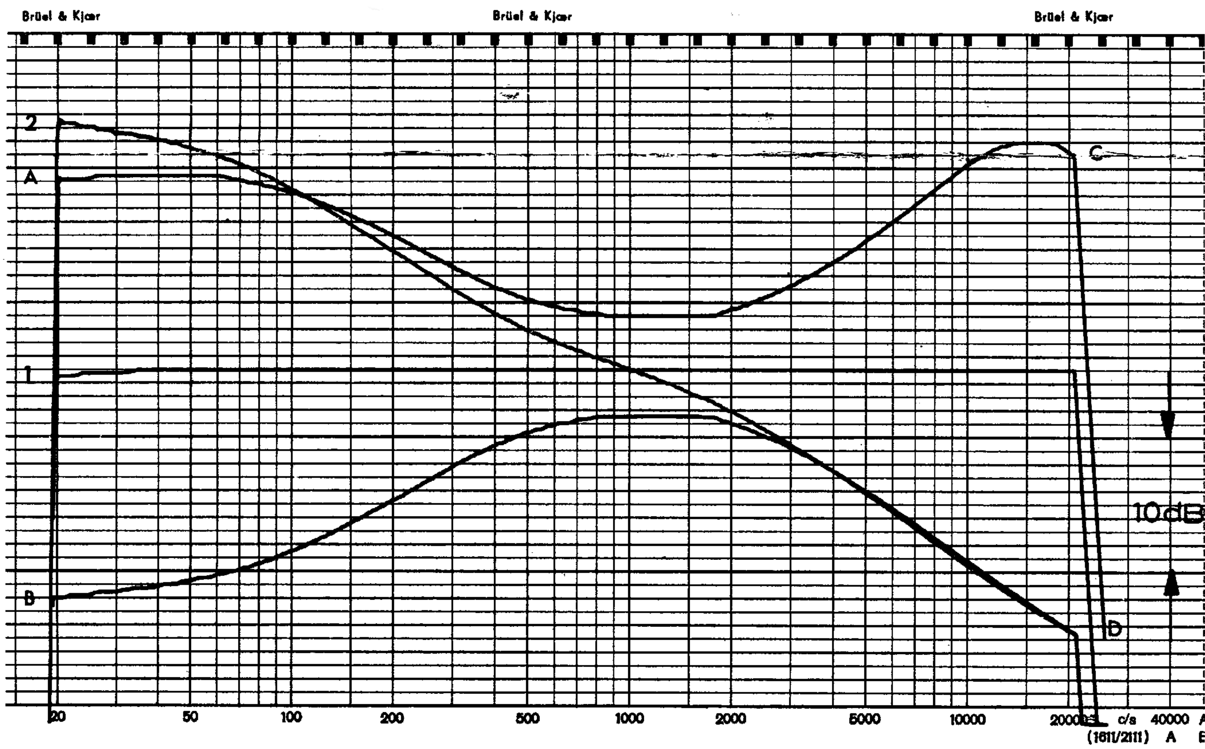
Frequenzgang 1 Eingänge RADIO, BAND 2 Phono-Entzerrung Wirkungsbereich der Klangregler A Bässe angehoben B Bässe abgesenkt C Höhen angehoben D Höhen abgesenkt
