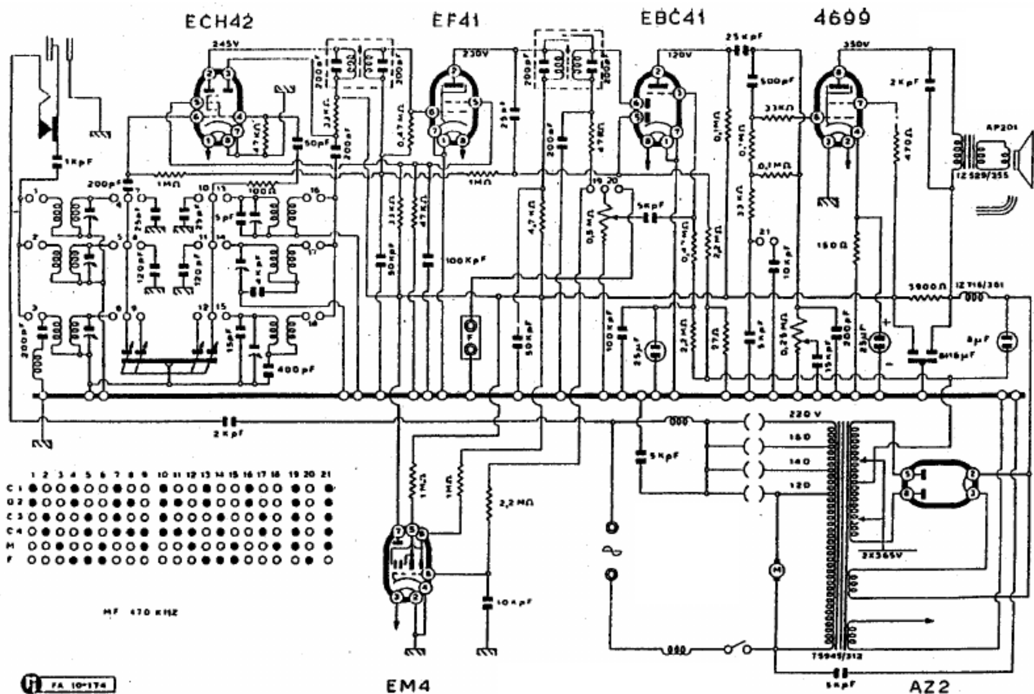
Kosmovox - Mod. 235, 935 Fono
