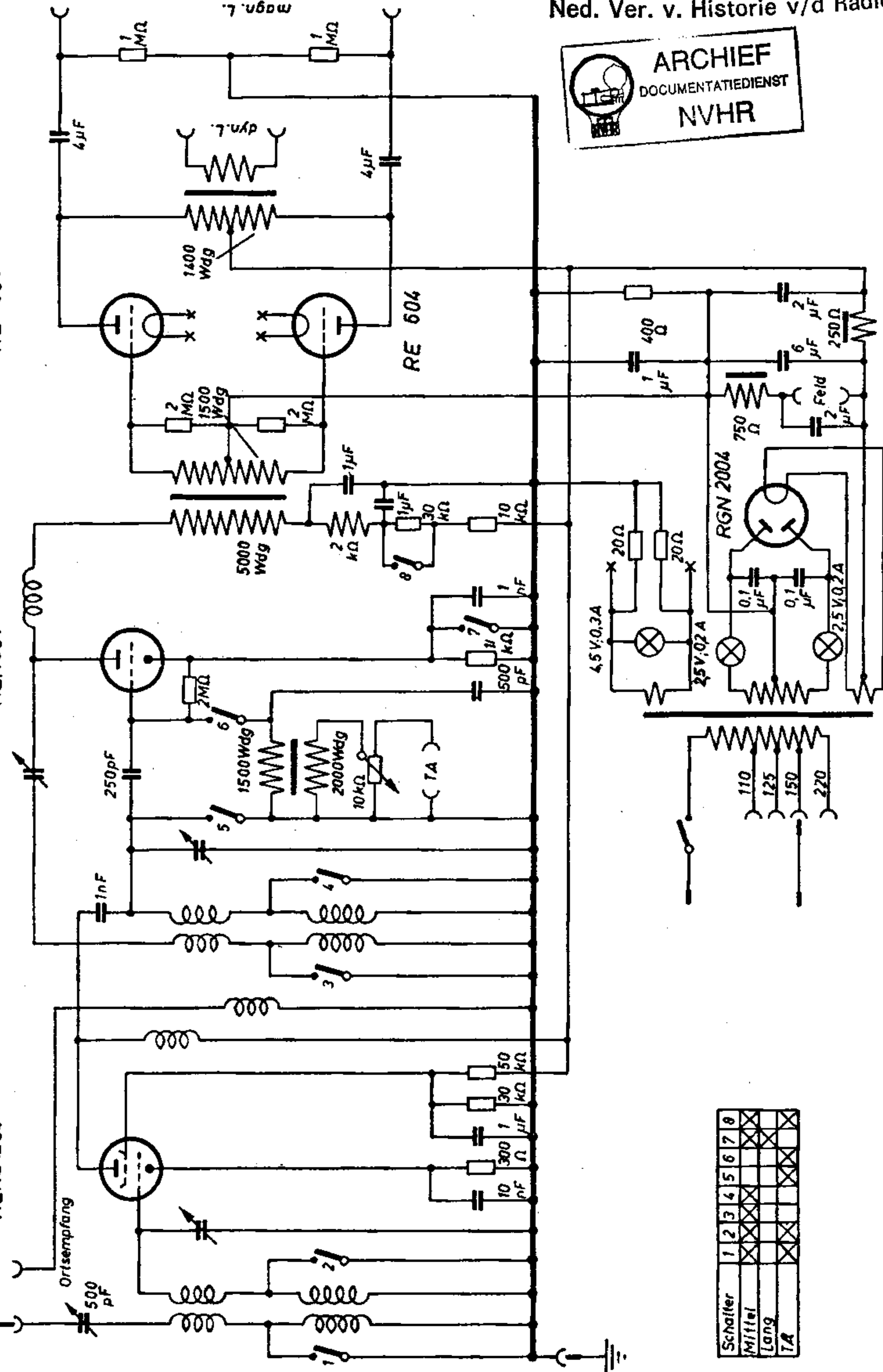
Lumophon RK 6 Roland
