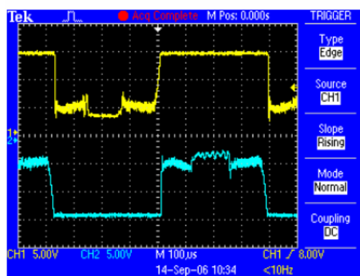
Clip 1.3 kHz.
