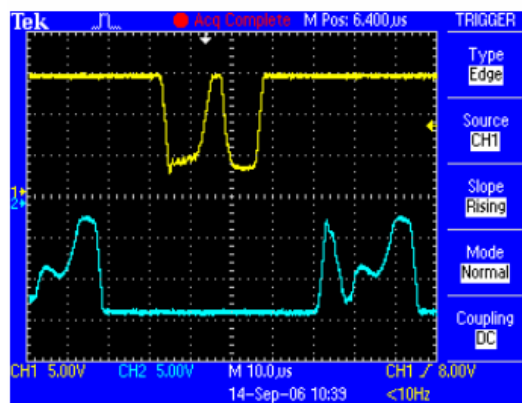
Clip 13 kHz.
