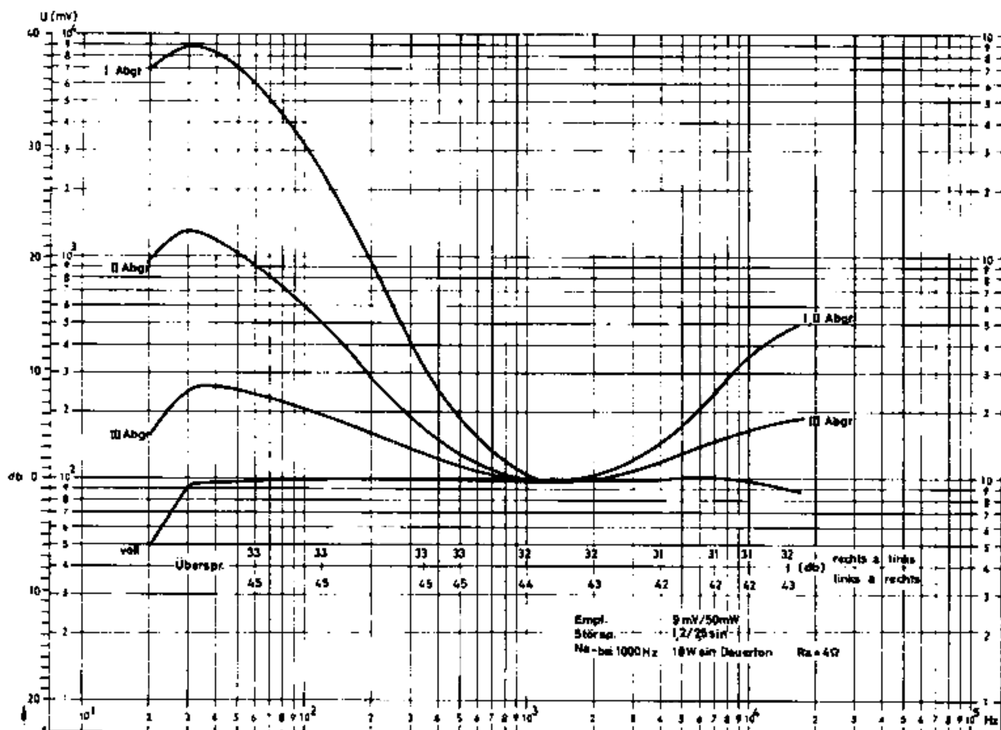
Bild 2: Frequenz-Kurven des NF-Verstärkers für verschiedene Lautstärkereger-Stellungen
