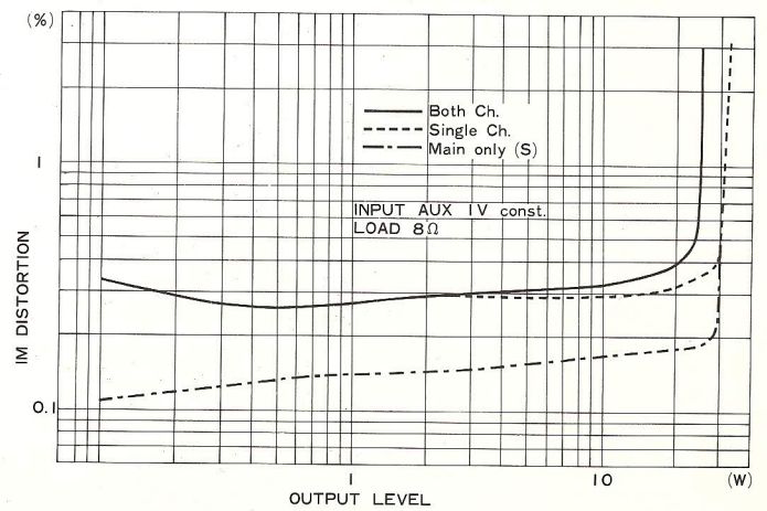
IM DISTORTION (70Hz : 7KHz) 4 : 1
