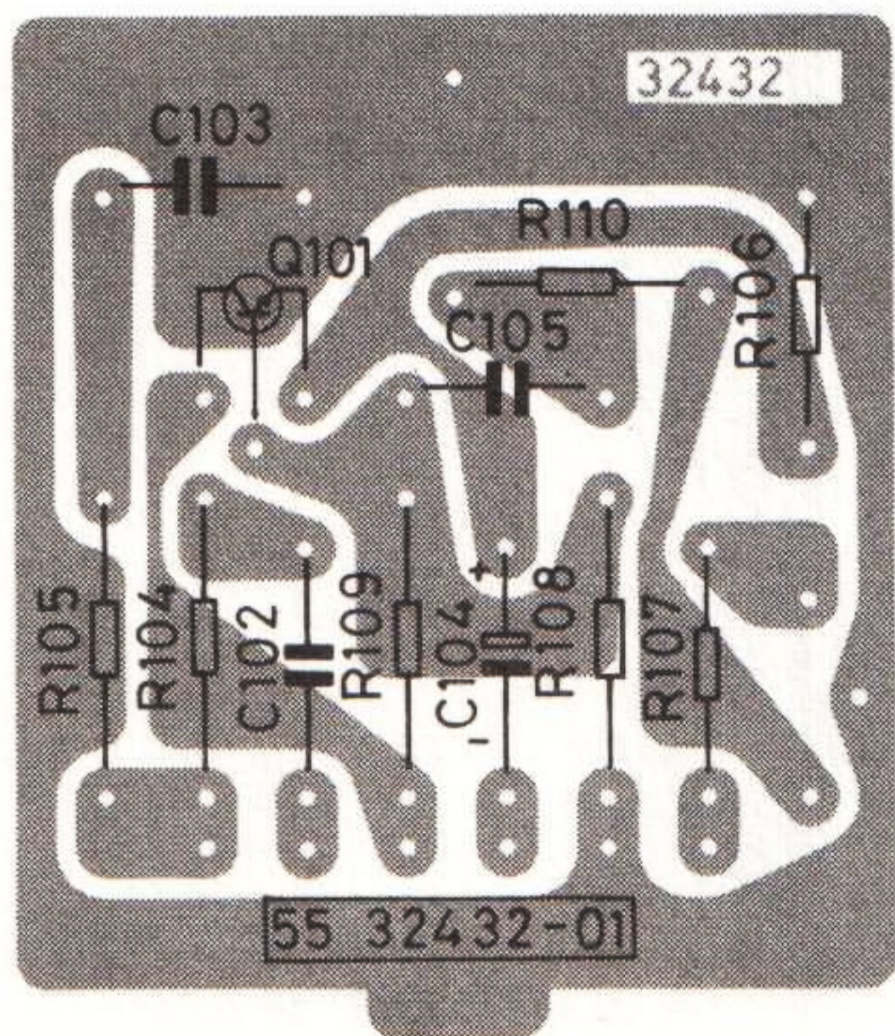
Foliesida
