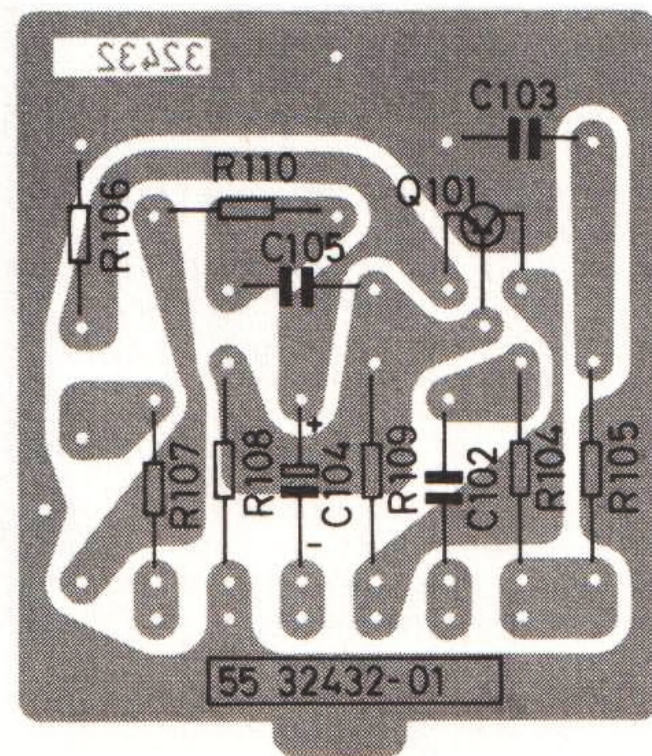
Komponentsida
