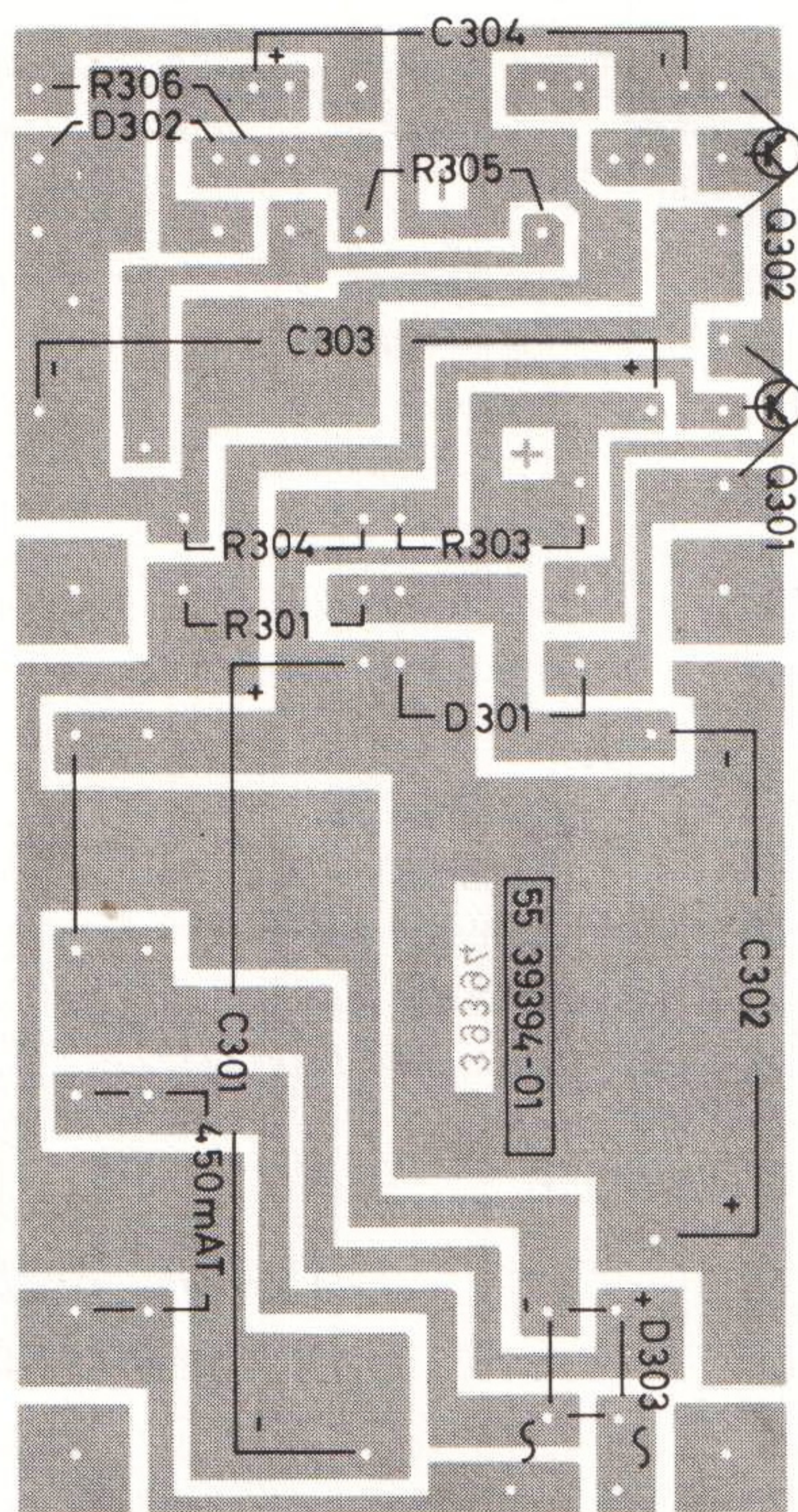
Komponentsida
