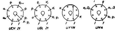
SOKKELFORBINDELSER
