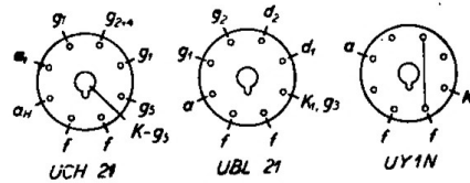
Sokkelforbindelser.
