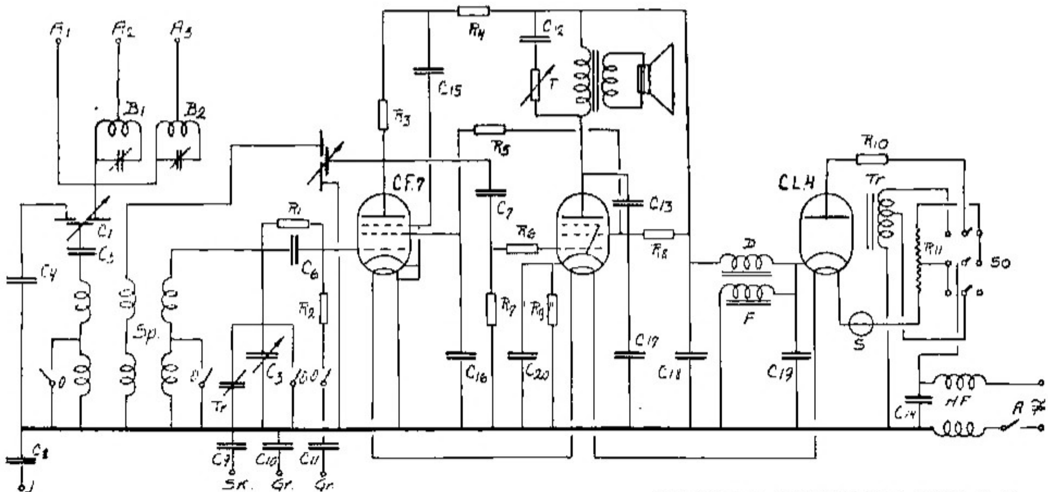
Diagrammet til Magnavox »Salon 37«.
