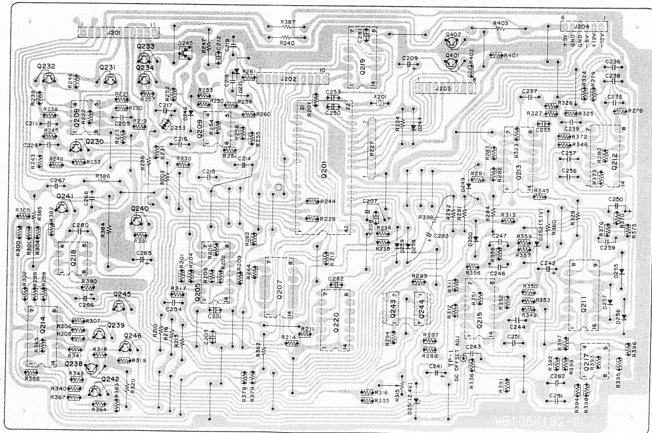
(P200) Servo
