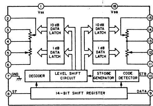
Q602 : TC9213P
