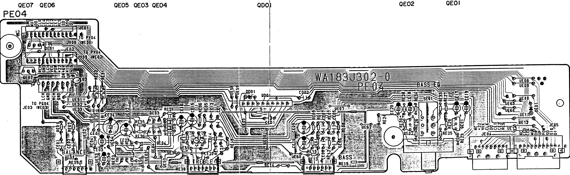
QD01 : LB1641
