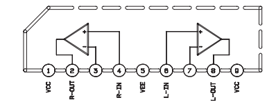
IC32 : MC4558S
