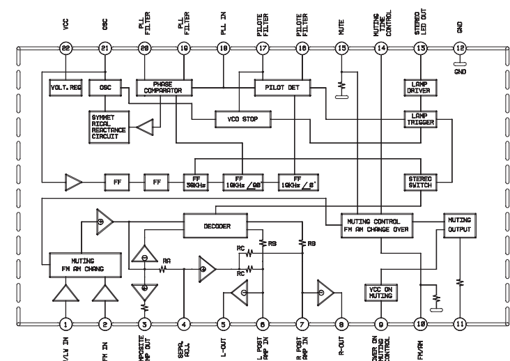
IC31 : LA3401
