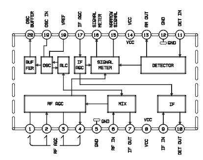
IC21 : LA1135
