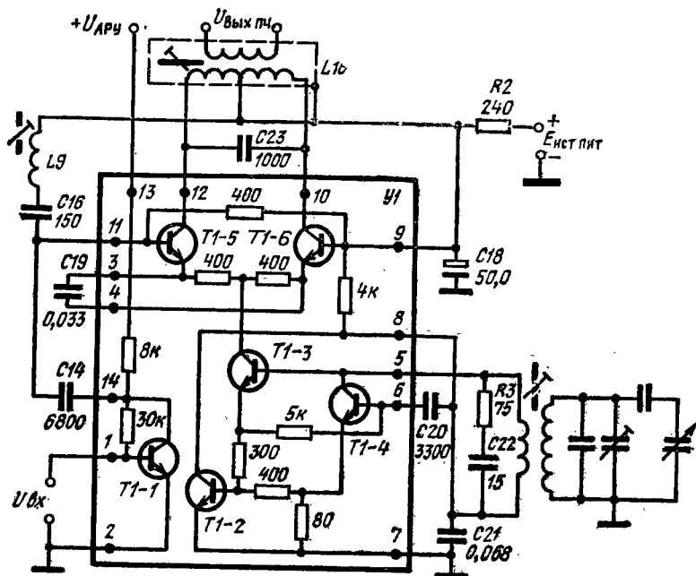
Принципиальная схема усилителя ВЧ, смесителя и гетеродина приемников «Украина-201» и «Меридиан-201».
