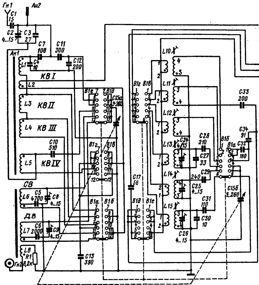
Принципиальная схема приемников «Украина-201» и «Меридиан-201».
