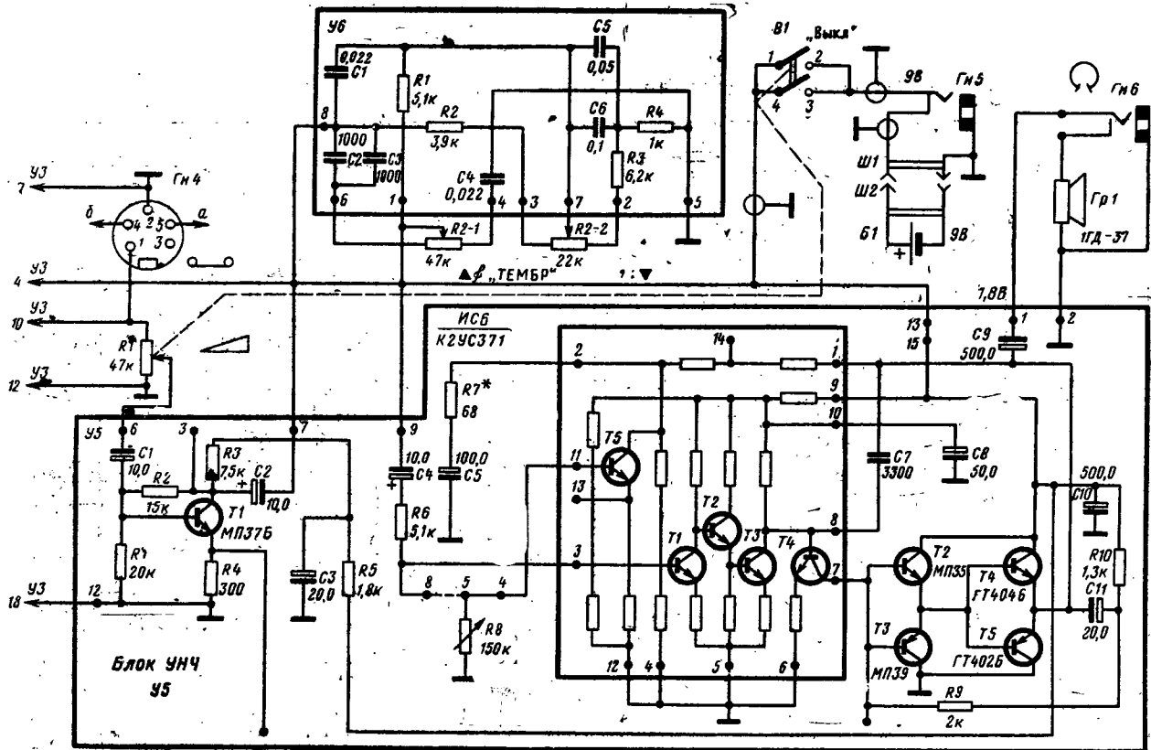
Принципиальная электрическая схема блока усилителя НЧ (У5) радиоприемника «Меридиан-206»
