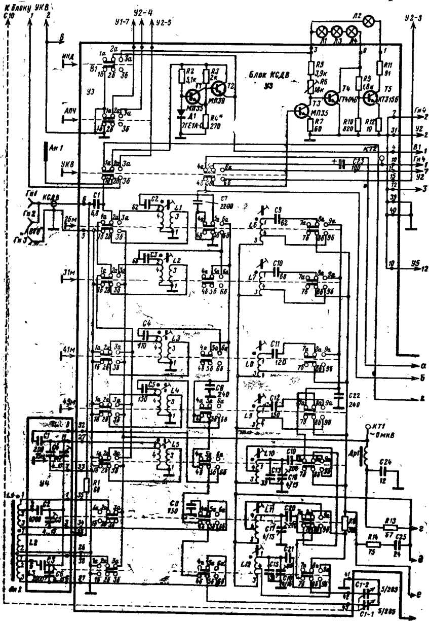
Принципиальная электрическая схема блока КСДВ (У3) радиоприемника «Меридиан-206»
