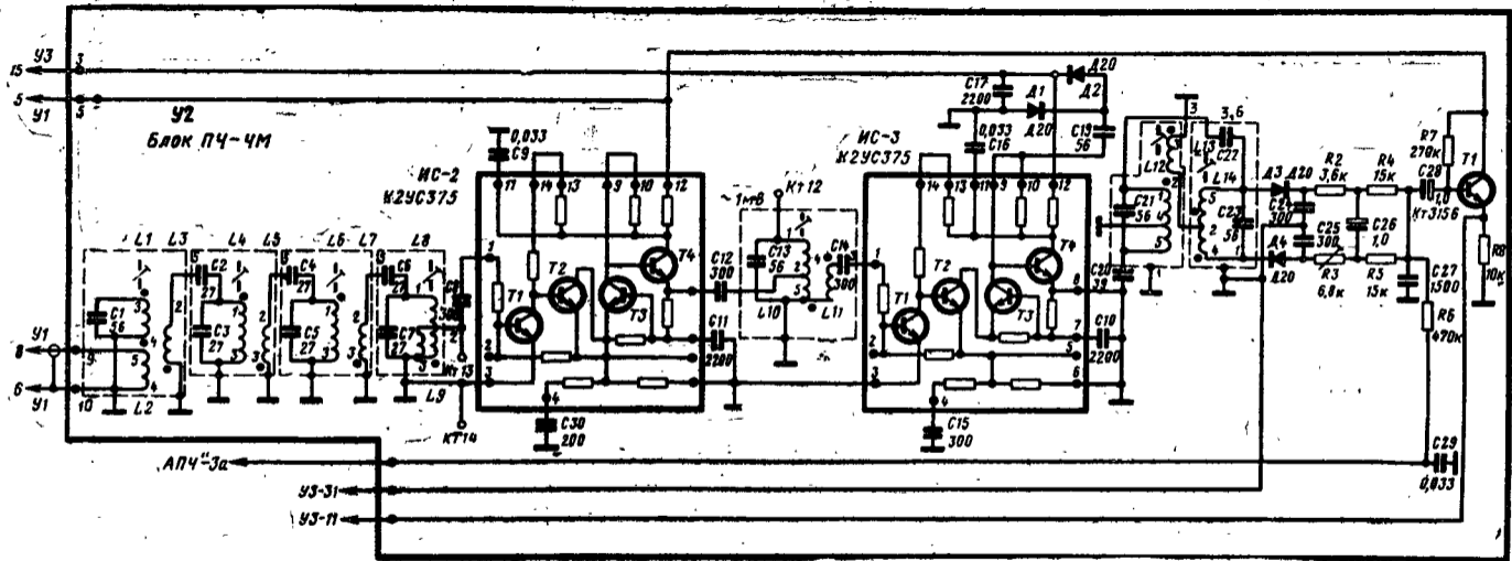
Принципиальная электрическая схема блока ПЧ-ЧМ (У2) радиоприемника «Меридиан-206»
