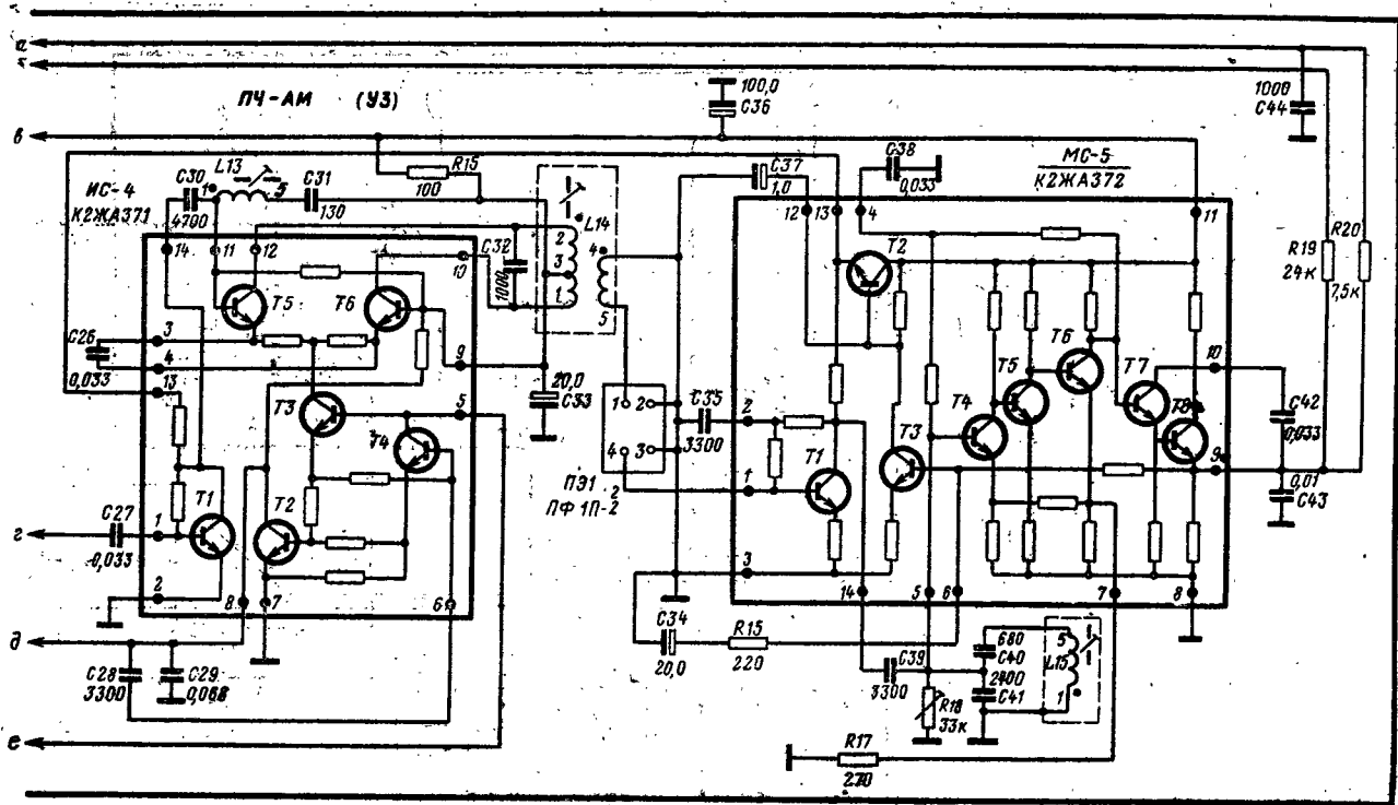
Принципиальная электрическая схема блока ПЧ-AM (У4) радиоприемника «Меридиан-206»
