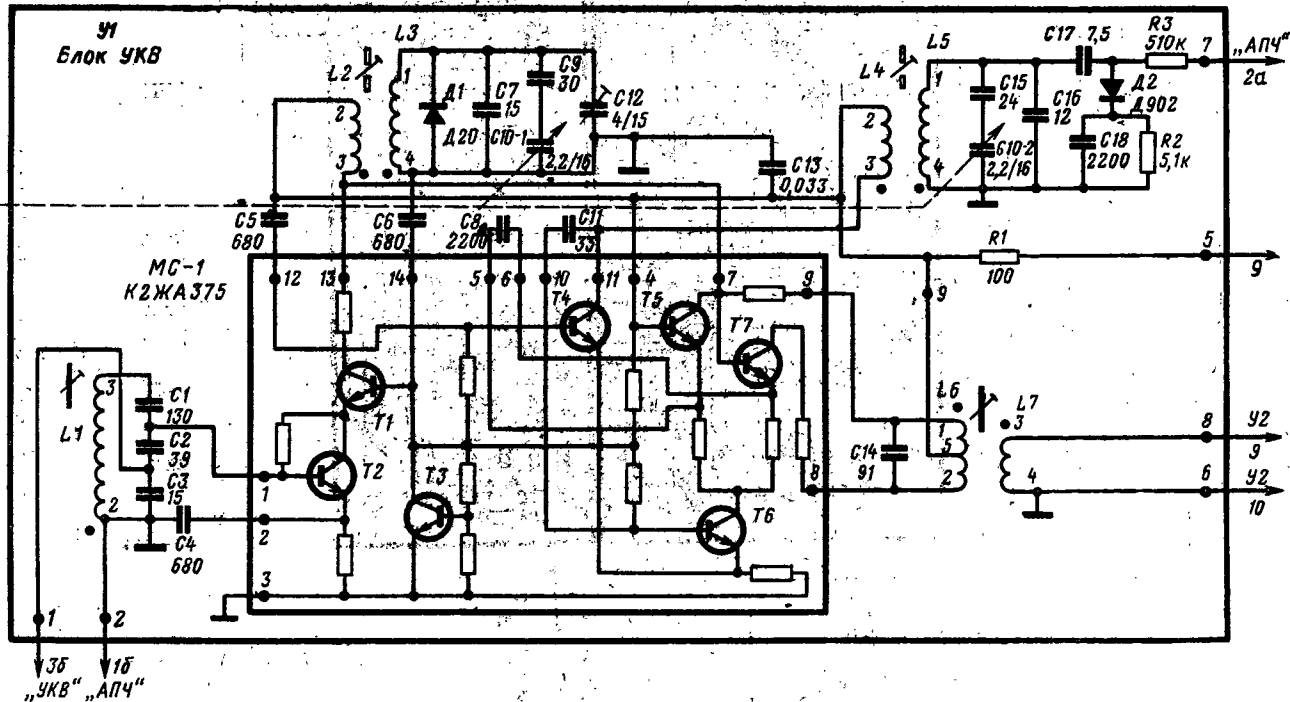
Принципиальная электрическая схема блока УКВ (У1) радиоприемника «Меридиан-206»
