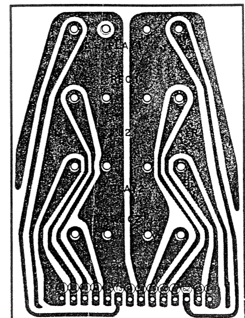
Tonbandgerät-Leiterplatte
