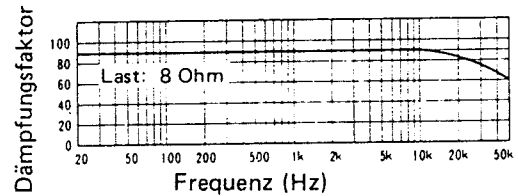
Dämpfungsfaktor
