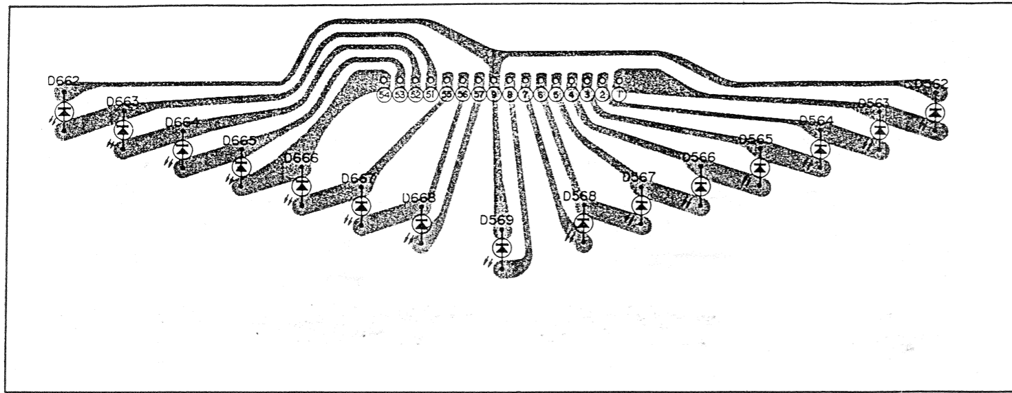
Anzeige-Leiterplatte
