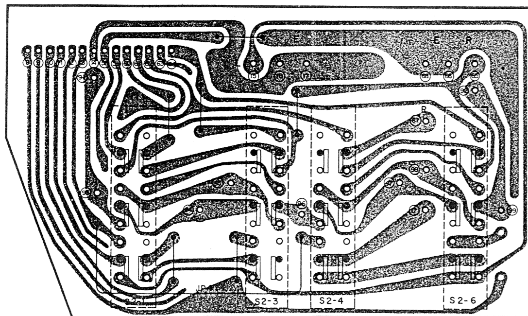
Kopierschaltungs-Leiterplatte
